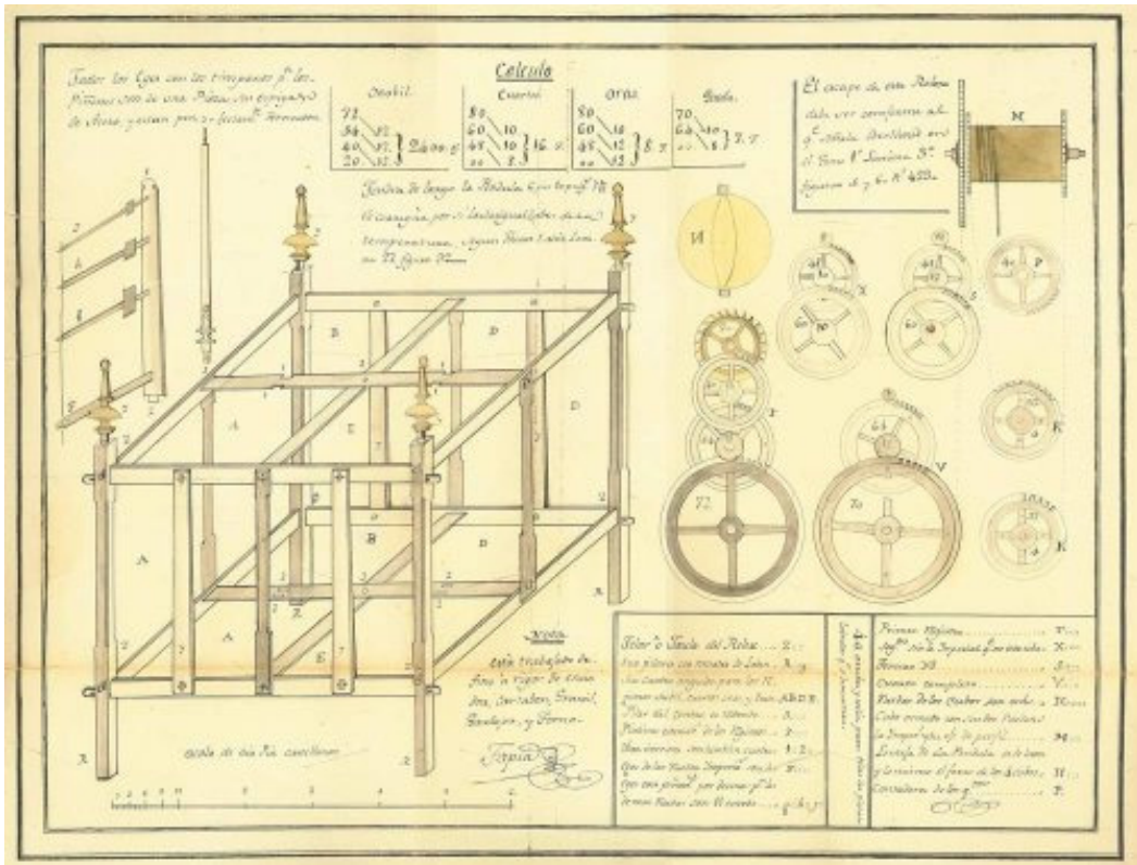
Planos del reloj del Ayuntamiento diseñados por Fernando de Tapia donde se muestra la estructura y engranajes de la maquinaria.
