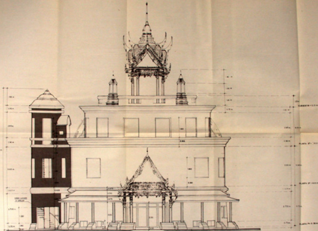
ALZADO 1
