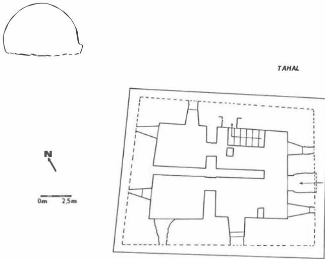
FIG. 7. Torre-castillo cristiana de Tahal: plano al nivel de la primera planta.
