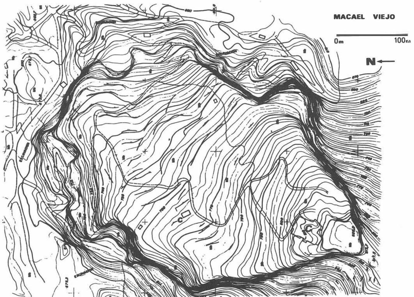
FIG. 5. Topografía del yacimiento de Macael Viejo. El despoblado medieval se extiende principalmente por la zona norte y noreste, mientras la zona de pendiente más fuerte, al suroeste, conserva vestigios de una necrópolis: c: aljibe; C: cantera moderna.
