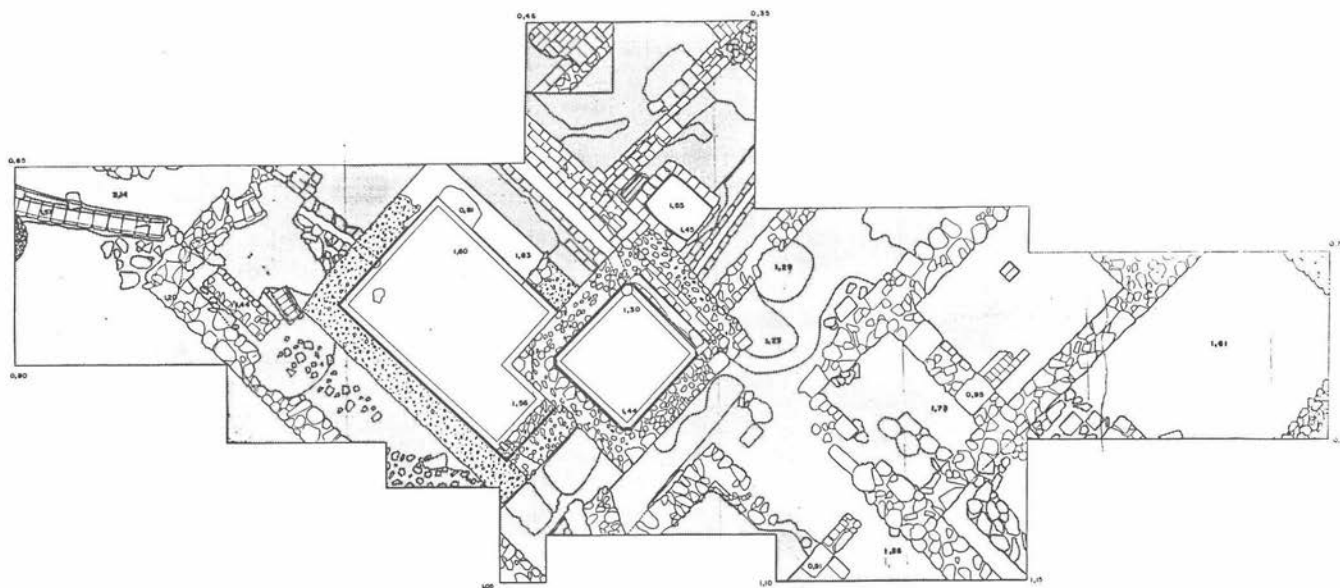
FIG. 1. Plantas.
