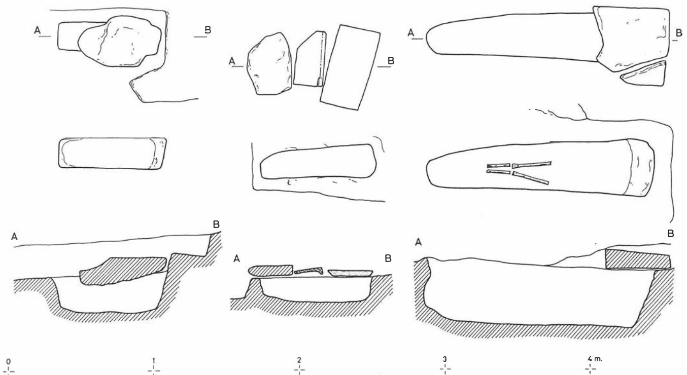
FIG. 1. Tumbas 1, 2 y 3. Plantas y secciones.
