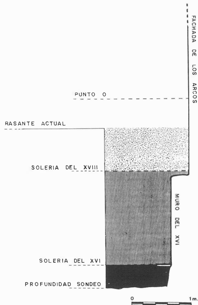
Fig. 3. Excavaciones Casa de la Moneda/86. Patio de los Capataces. Corte 2 Sección A-B.
