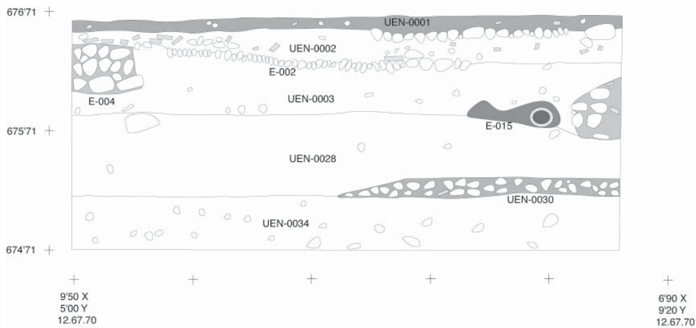
FIG. 2. Sección sector 1.
