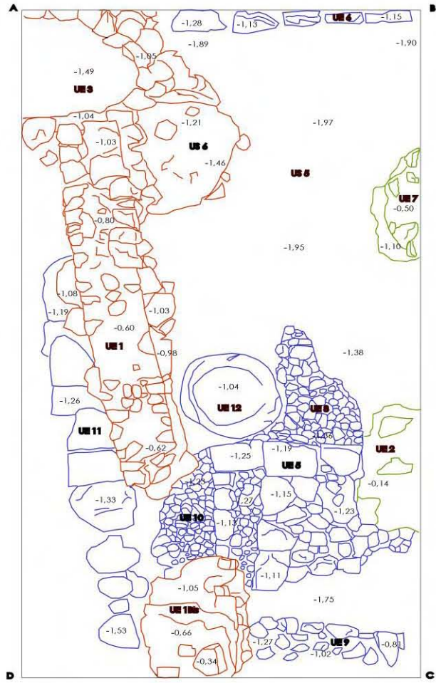
Piano 3/3. PLANTA GENERAL DE LA EXCAVACIÓN
