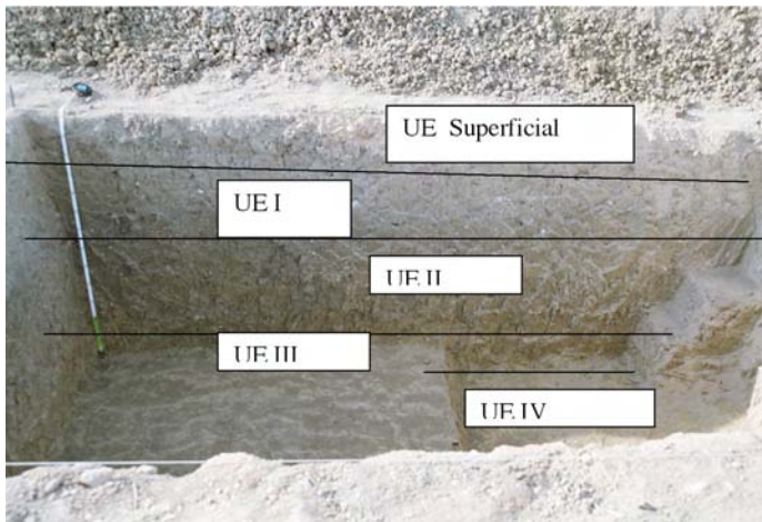
Lámina II. Perfil estratigráfico Oeste del Corte 1
