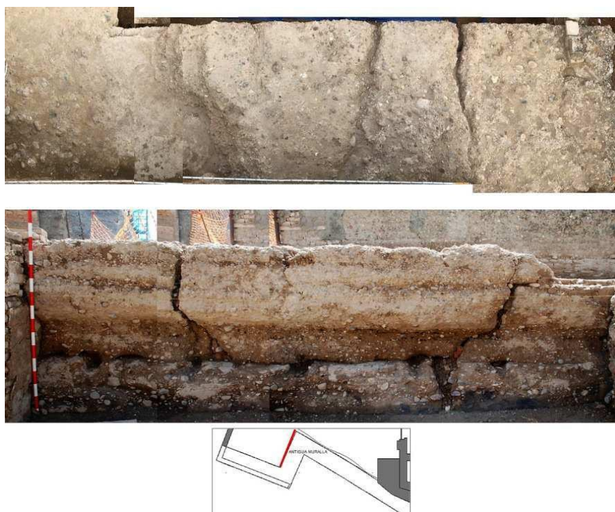
FIGURA 4. Planta y alzado del tramo 2 de la muralla.
