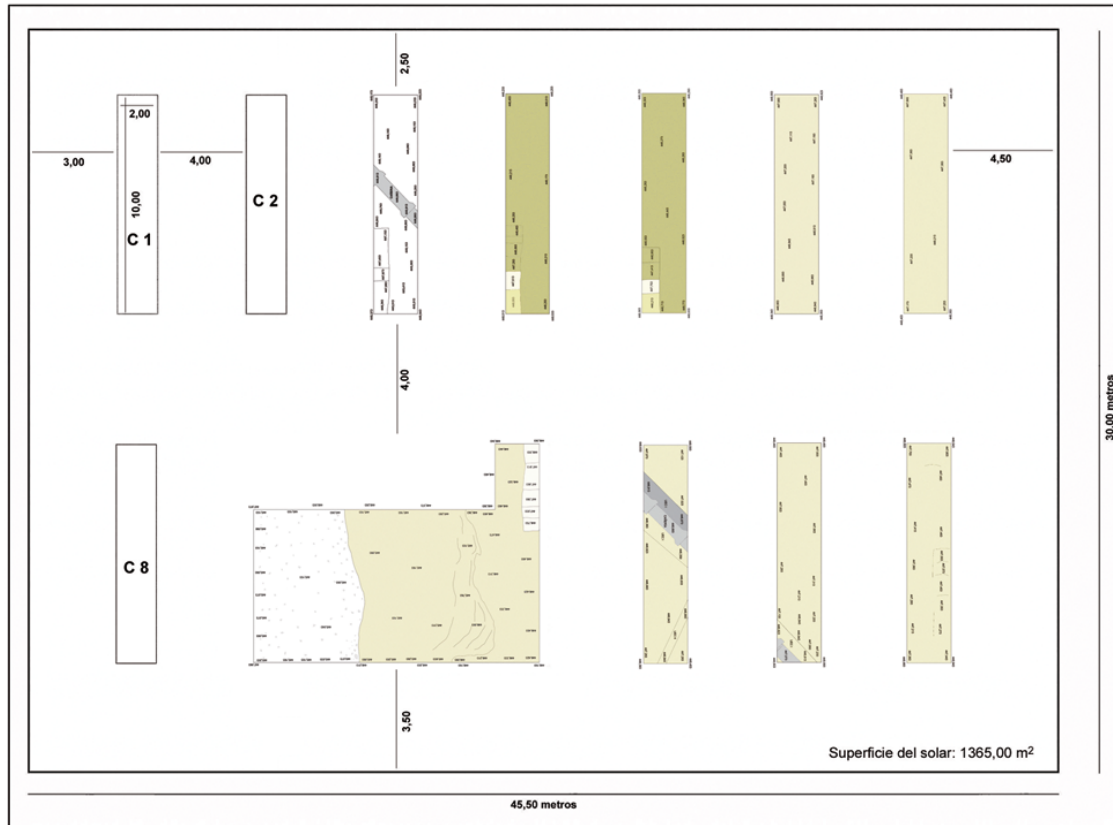
FIG. 2: Planteamiento de la excavación.
