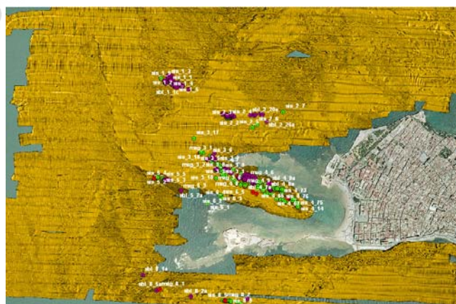
Fig 2. Mosaico a partir del registro de sonar con los puntos de anomalías.
