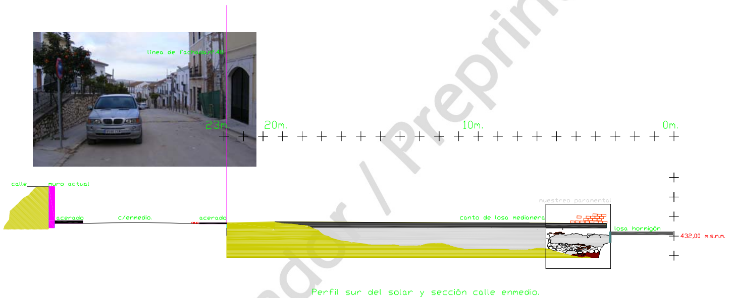
Fig.1. Perfil longitudinal del solar nº 48 en relación a la calle enmedio.
