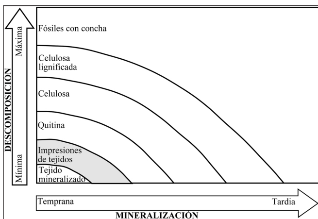
FIG. 10: Diagrama que muestra la relación entre la descomposición y la mineralización en la preservación de organismos de cuerpo blando y/o debilmente esqueletizados (modificado de Allison, 1988, 1990). La zona oscurecida señala la situación (hasta el momento) de los fósiles del K. F.-L. de Cuevas de Almazora. La posible existencia de tejido mineralizado está en estudio.
