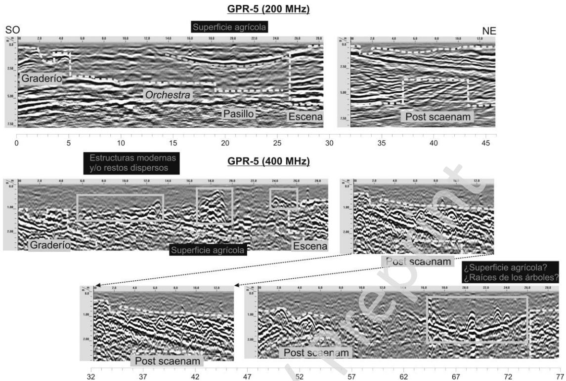
Figura 20. Radargrama de la sección GPR-5.
