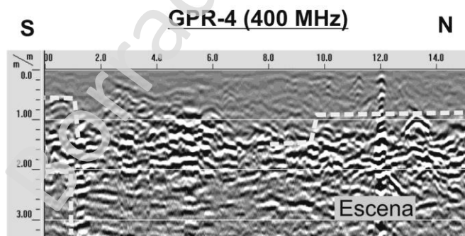
Figura 21. Radargramas de las secciones GPR-4 y GPR-6.
