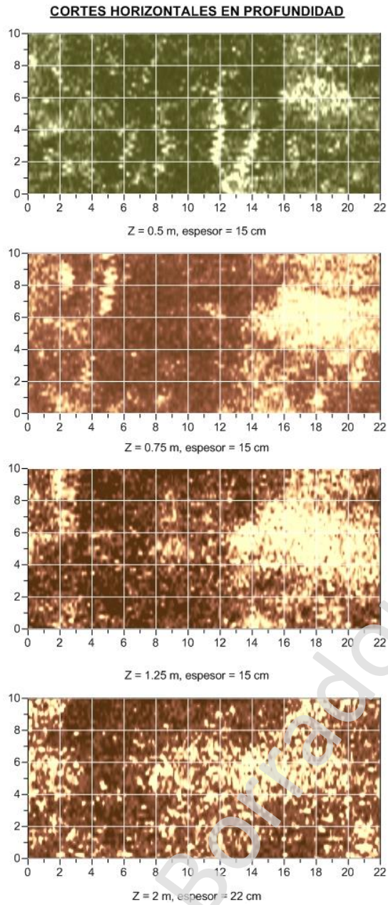
Figura 18. Cortes horizontales obtenidos a partir de la exploración con georradar del sector RADAR-3.
