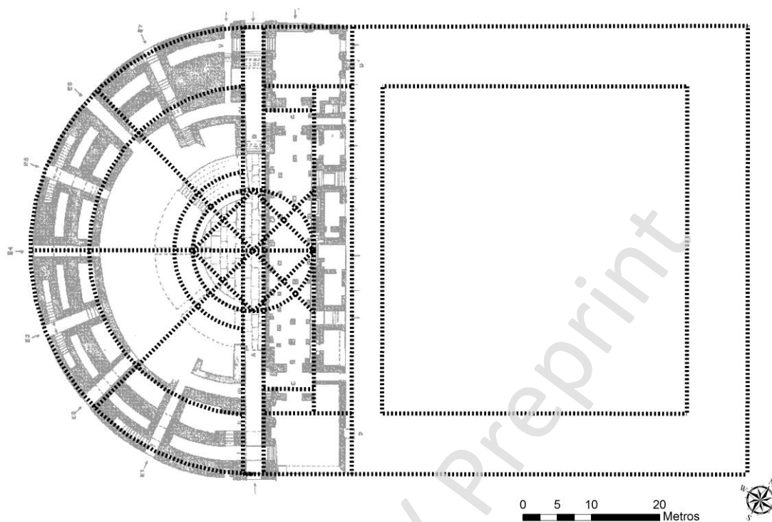
Figura 25. Esquema geométrico del teatro romano de Osuna (línea discontinua gruesa) superpuesta sobre la planta del anfiteatro romano de Baelo Claudia (Jansen, 2005, fig. 7).
