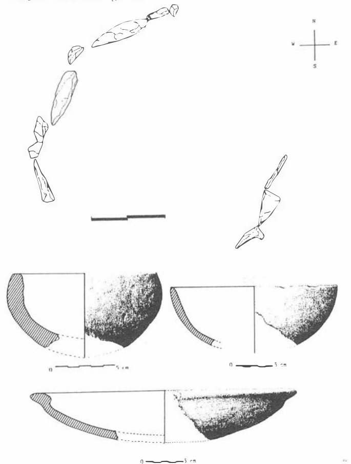
FIG. 3. Dolmen de Los Delgados IV.
