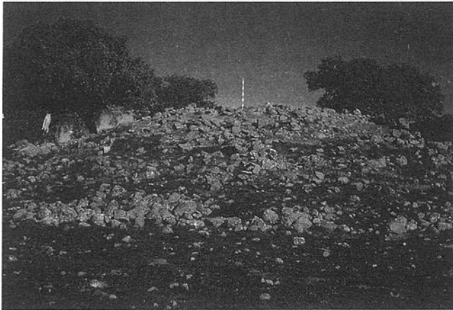
LAM. III. Túmulo del Dolmen de La Sierrezuela I.
