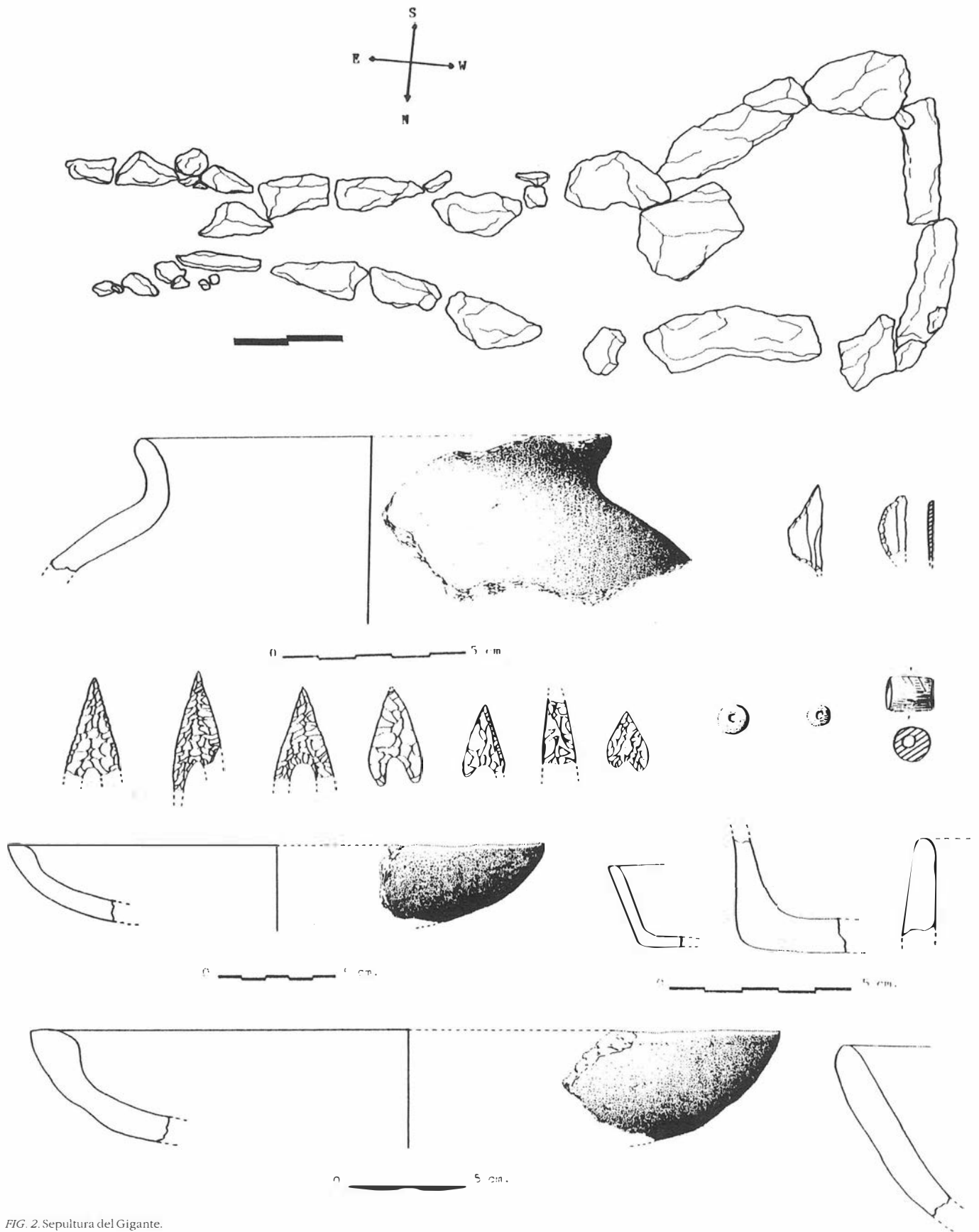
FIG. 2. Sepultura del Gigante.
