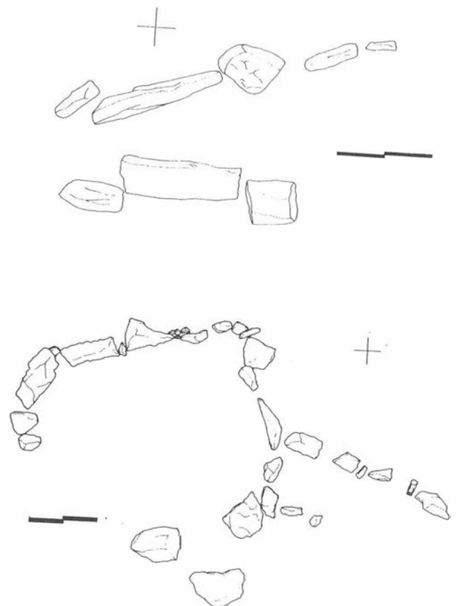
FIG. 5. A) Dolmen de Doña Rama I. B) Dolmen de La Horma.
