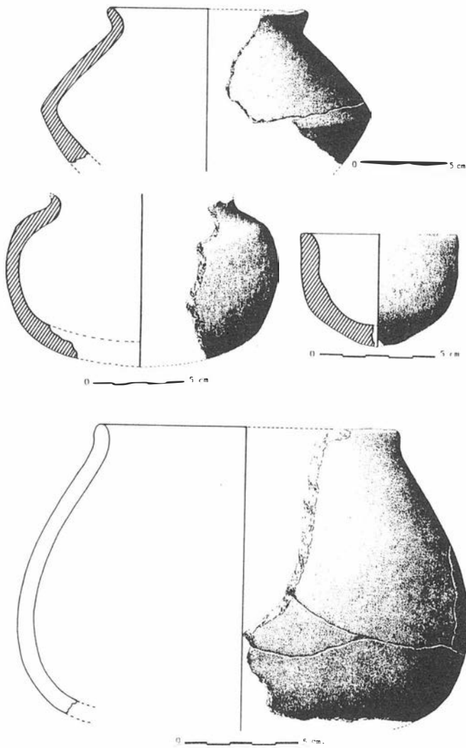
FIG. 4. Dolmen de Los Delgados IV.
