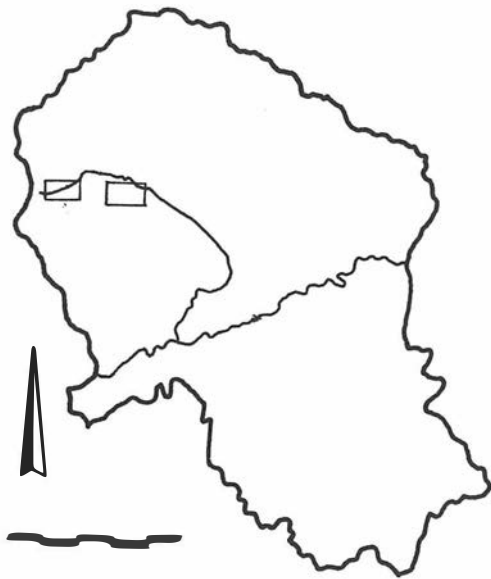
FIG. 1. Localización de las sepulturas megalíticas.
