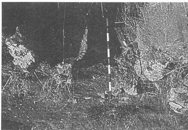
LAM. IIIa. Sepultura del Gigante. LAM. IIIb. Dolmen de La Horma.
