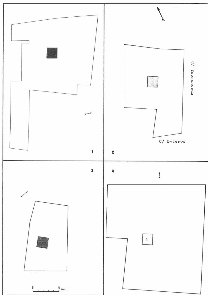
FIG. 2. Planos de los solares de c/ Alhóndiga, nº 24 (1), c/ Boteros, nº 27 (2), c/ Céspedes, nº 9 (3), c/ Bécquer, nº 37 (4), con indicación de los sondeos efectuados.
