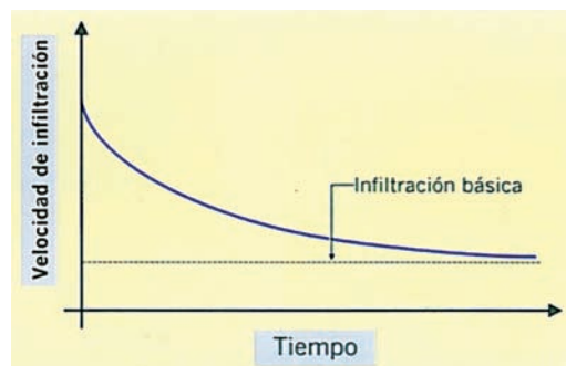
Figura 9. Curva que refleja la variación de la infiltración del agua en un suelo a medida que pasa el tiempo.
