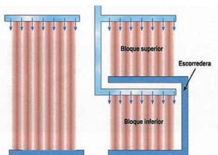
Figura 9. Diseño de la parcela de riego en bloques independientes cuando se decide acortar la longitud de los surcos o las fajas.
