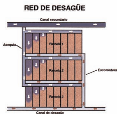
Figura 7. Esquema de escorrederas y red de desagüe.
