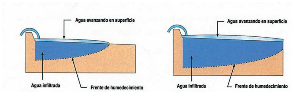
Figura 11. Perfil del agua infiltrada durante el avance y durante el humedecimiento del suelo.
