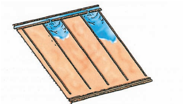
Figura 5. Riego por fajas, con acequia de abastecimiento en la cabecera y desagüe en cola.
