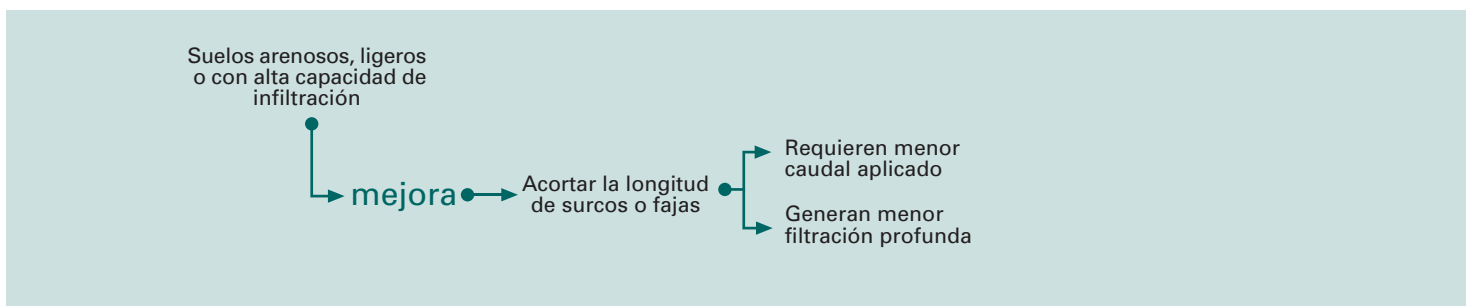
Figura 8. Efectos de la reducción de la longitud de las unidades de riego en suelos ligeros con alta capacidad de infiltración de agua.
