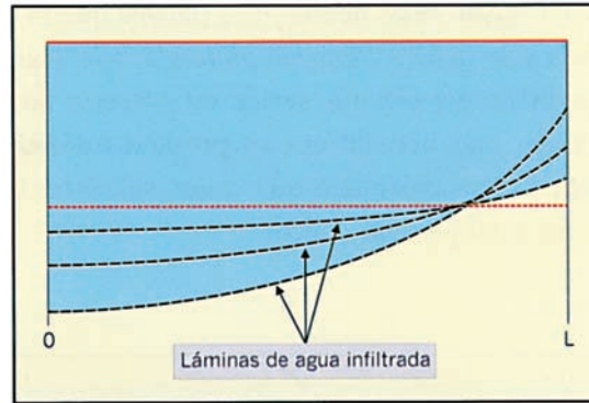
Figura 6. Respetando el mismo criterio de diseño se pueden conseguir diferentes uniformidades de aplicación.
