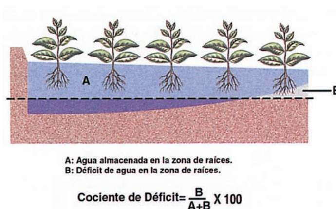
Figura 1. Representación esquemática de los elementos que intervienen en el cálculo del cociente de déficit.
