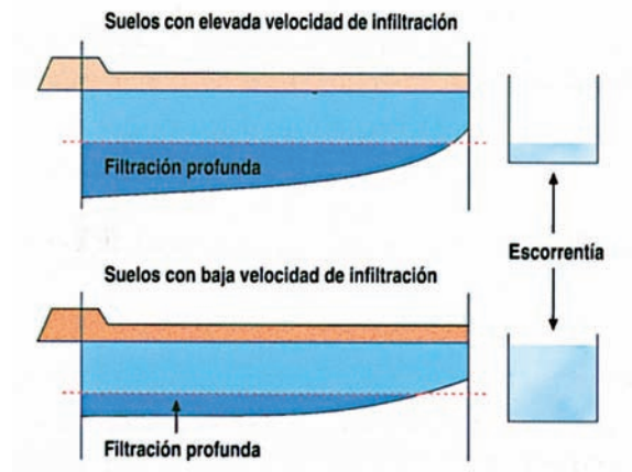
Figura 8. Pérdidas de agua por filtración profunda o percolación y por escorrentía según la velocidad de infiltración del suelo.
