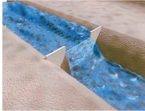
Figura 18. Vertedero rectangular.
