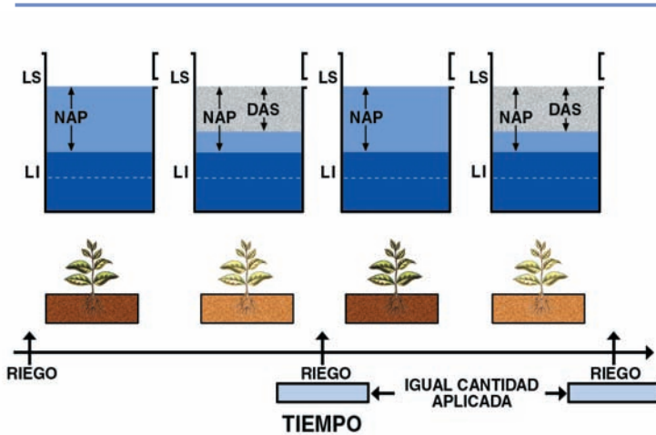
Figura 11. Estrategia de riego con la que se aplica una cantidad de agua fija
