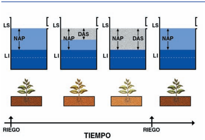
Figura 10. Estrategia de riego basada en aplicar las necesidades brutas cuando el DAS alcance el NAP
