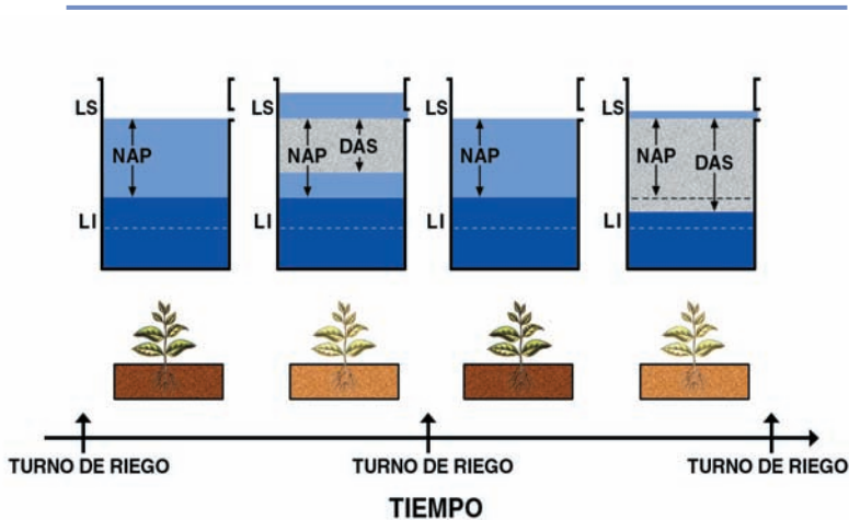
Figura 12. Riego establecido por turnos
