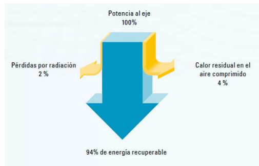
Figura 4. Desglose de energía en sistemas de aire comprimido.
