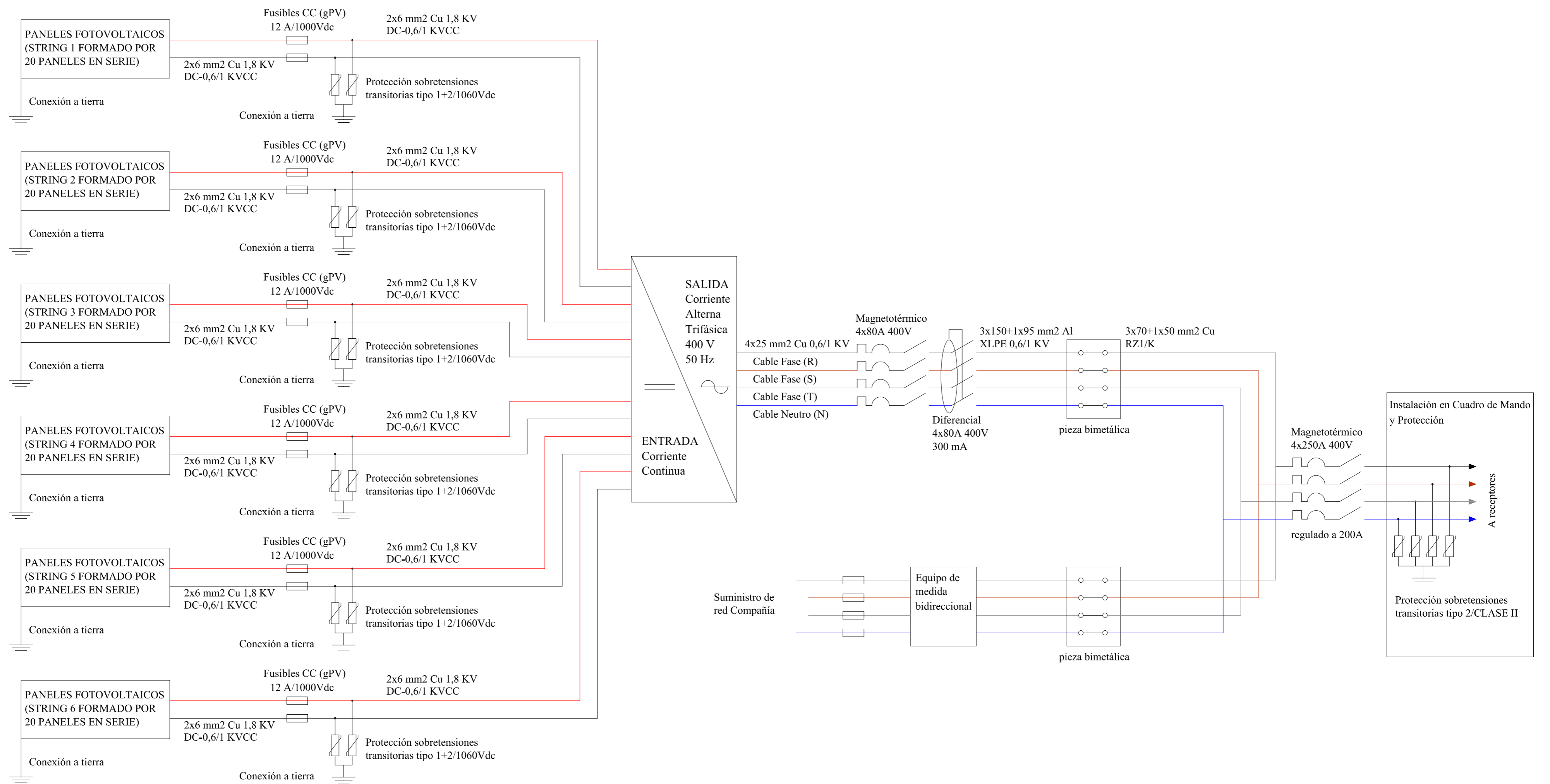
ESQUEMA UNIFILAR
