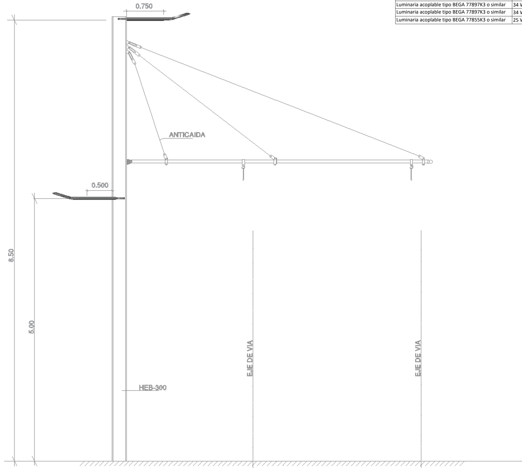
EQUIPO CON PALANCAS, CON POSTE FUERA DE LA ENTREVIA, PARA VIA DOBLE EN CURVA DE RADIOO <1500m,
