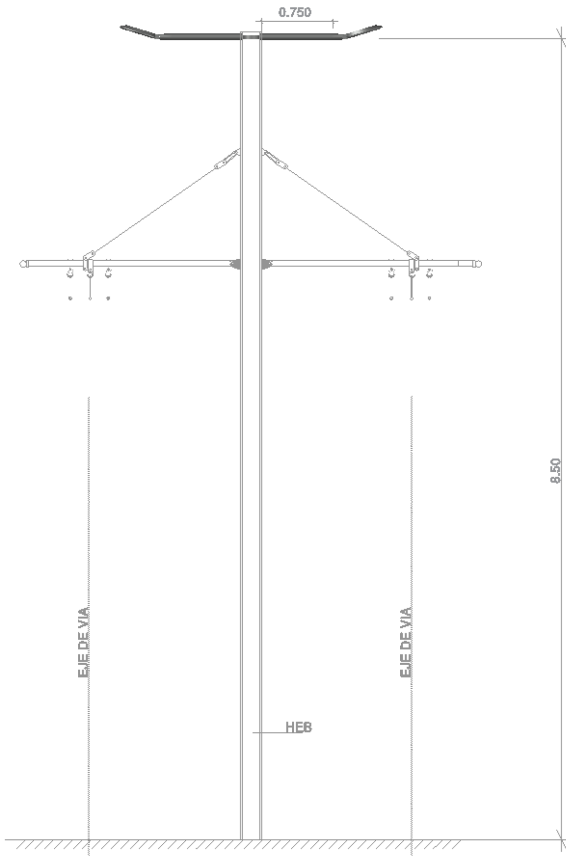
EQUIPO PARA VIA DOBLE EN RECTA Y CURVA DE RADIO >1500m.
