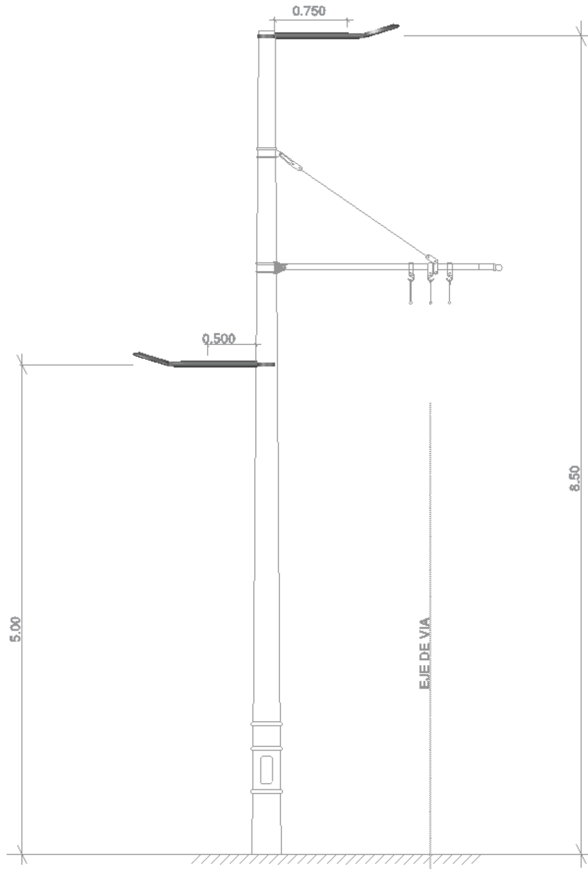
EQUIPO PARA VIA ÚNICA EN RECTA Y CURVA DE RADIO >1500m. CON POSTE DE ALTURA DE 8.50 ó 10.50m
