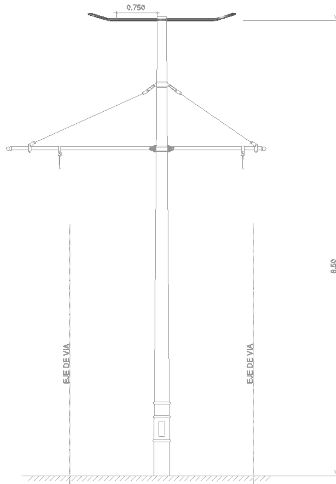
EQUIPO CON PALANCAS PARA VIA DOBLE EN CURVA DE RADIO <1500m. CON POSTE DE ALTURA DE 8.50 ó 10.50m
