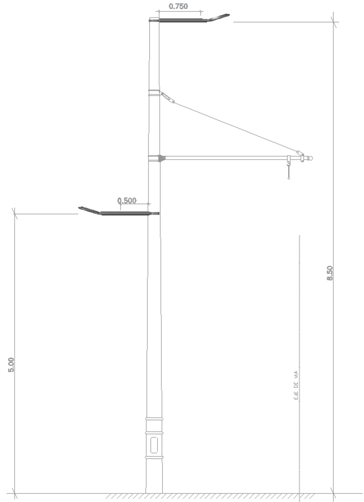
EQUIPO CON PALANCAS PARA VIA ÚNICA EN CURVA DE RADIO <1500m. CON POSTE DE ALTURA DE 8.50 ó 10.50m
