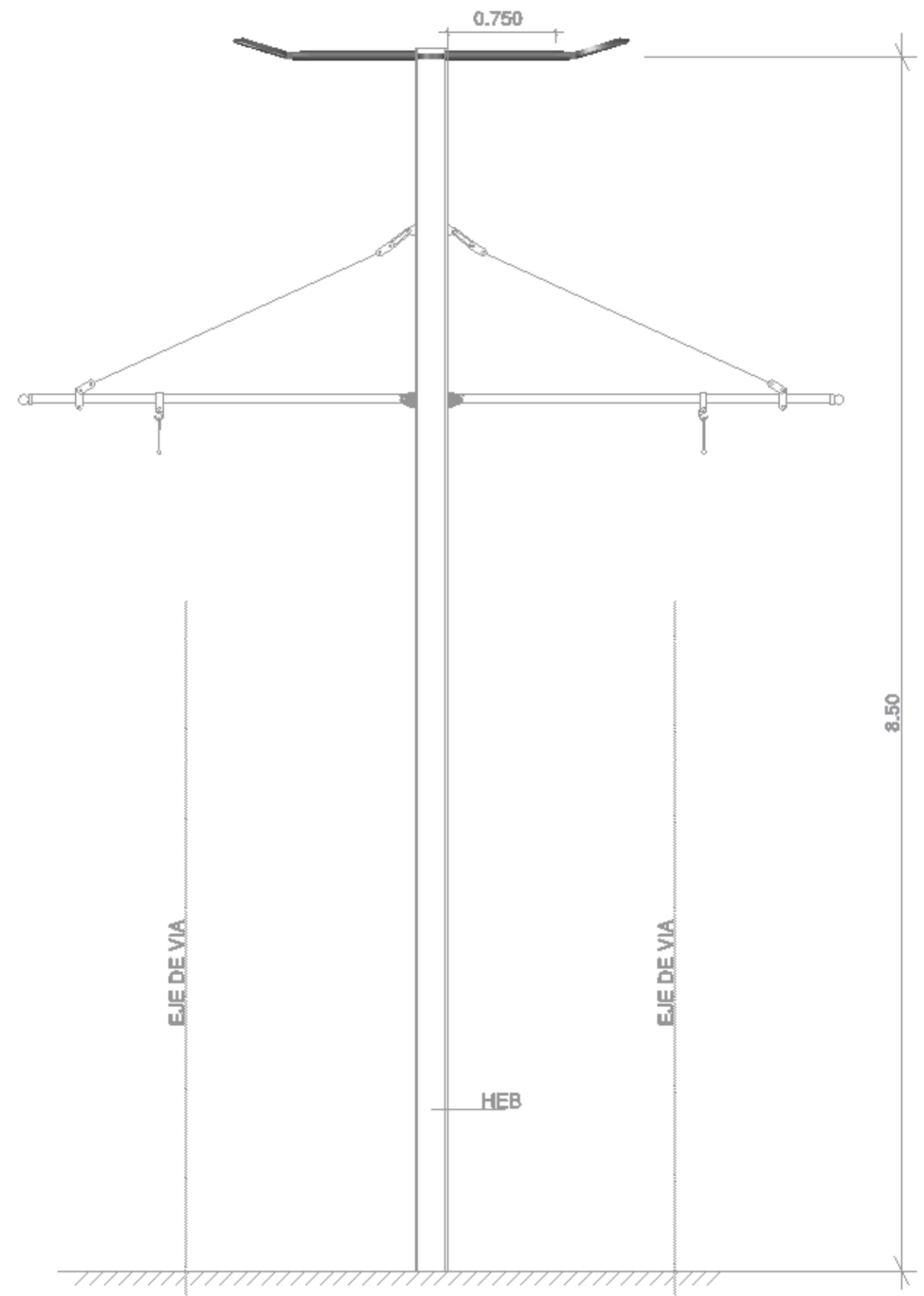
EQUIPO CON PALANCAS PARA VIA DOBLE EN CURVA DE RADIO <1500m.
