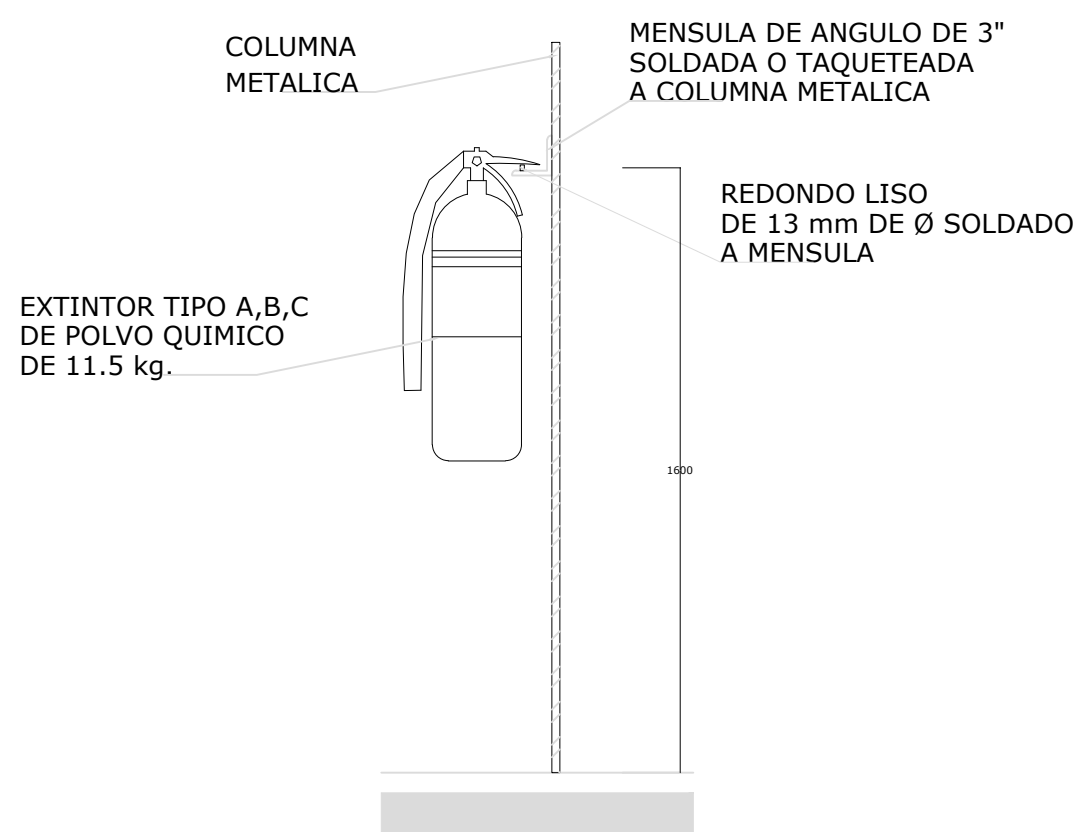
DETALLES CONTRA INCENDIOS ESC 1:20
