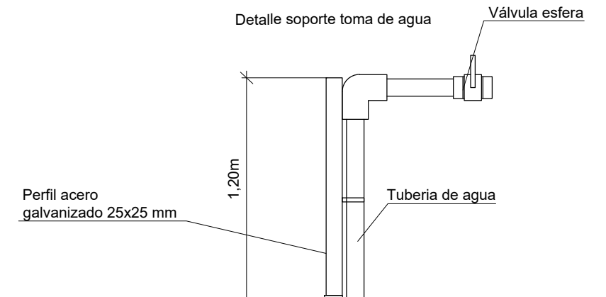
DETALLE TOMA DE AGUA COCHERA
