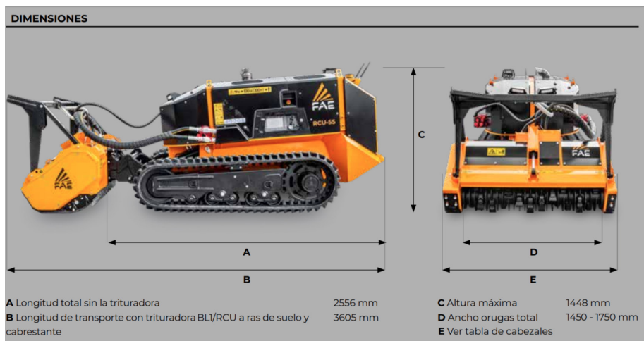
Imagen 1: Medidas cabeza tractora y cabezal desbroce (*)
