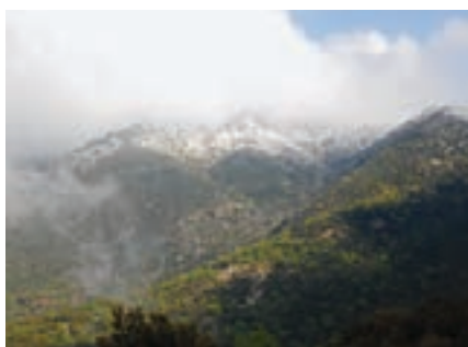
Nubes atrapadas en la sierra (efecto Foehn)
