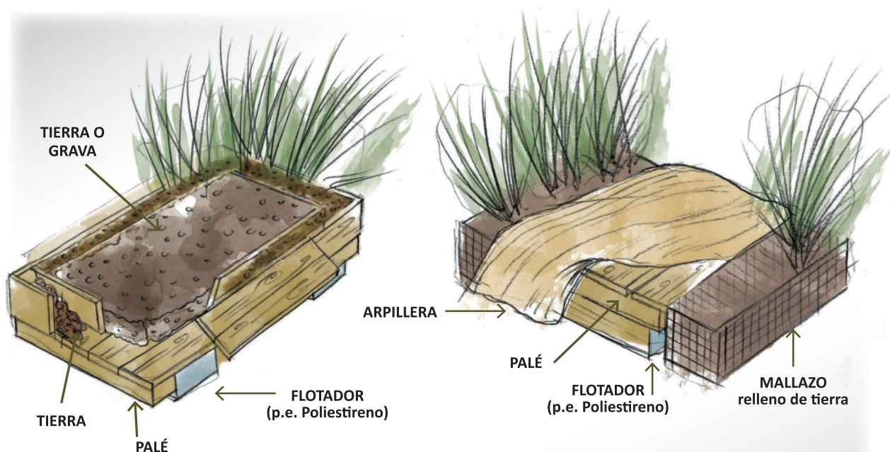
Figura 7. Ejemplos de construcción de isletas flotantes para ubicar en una balsa o charca natural o artificial. Fuente: Elaboración propia a partir de Camacho y col., (2011).
