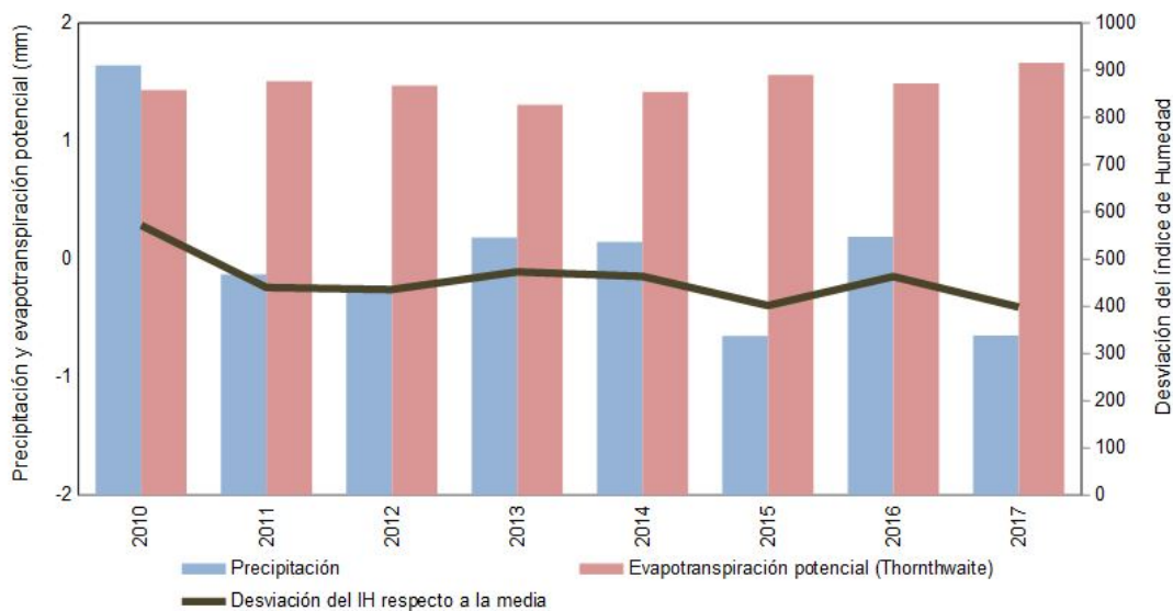
Precipitación, evapotranspiración potencial e índice de Humedad en Andalucía, 2010-2017
