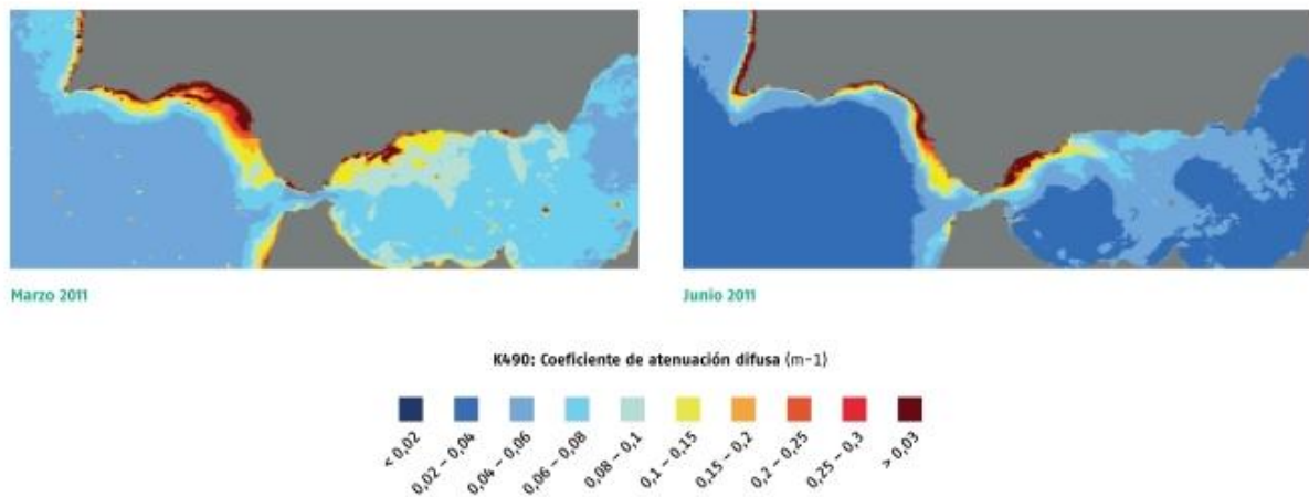
CONCENTRACIÓN MEDIA DE K-490 2011 A PARTIR DE IMÁGENES DE SATÉLITE AQUA-MODIS
