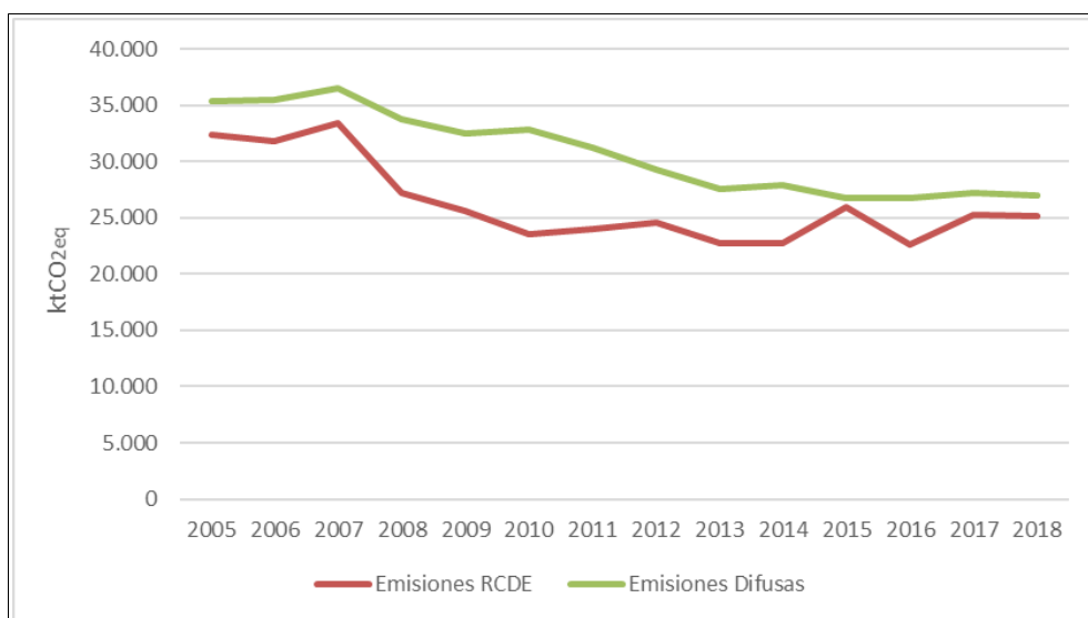
Figura 6. Evolución de las emisiones difusas y del RCDE en Andalucía
