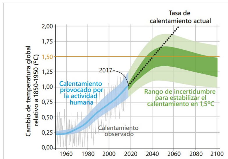
Figura 5. Calentamiento global inducido por el hombre
