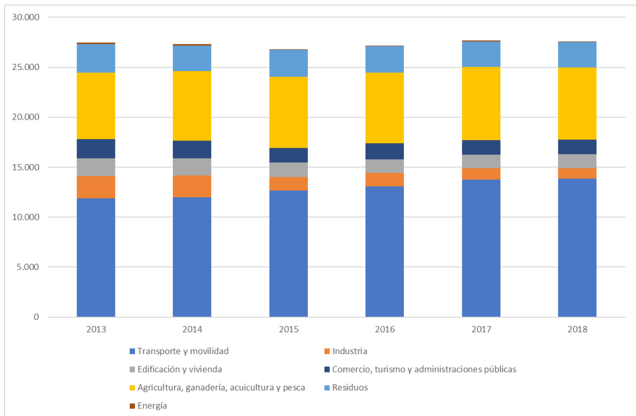
Figura 7. Evolución de las emisiones difusas de Andalucía por área estratégica (KtCO 2-eq )
