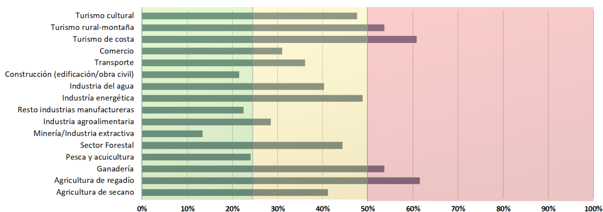
Figura 13. Evaluación del riesgo de los principales sectores económicos.
