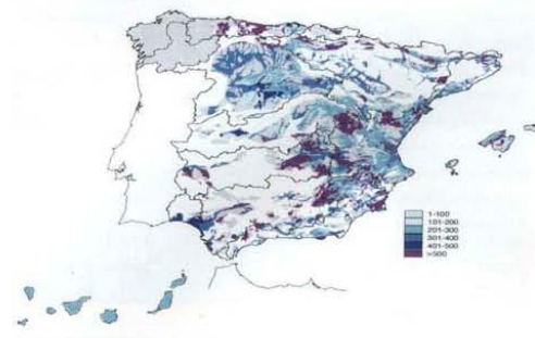
Figura 18. Mapa de capacidad de infiltración máxima (mm)
