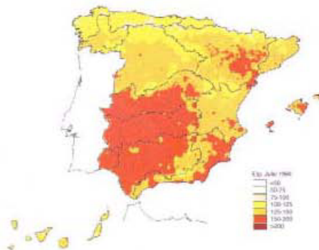
Figura 11. Cálculo de la ETP (mm) según Thornthwaite (julio 1990)
