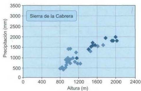
Figura 6. Establecimiento de regresiones precipitación-altura
