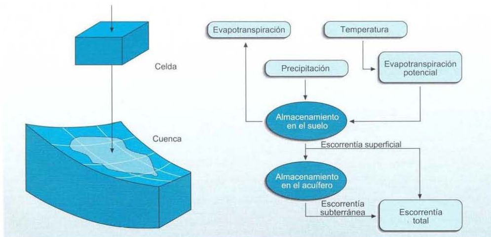
Figura 1. Diagrama de flujo del modelo distribuido SIMPA
