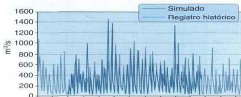
Figura 29. Series mensuales simuladas e históricas del río Ebro en Castejón (periodo 1940-1995)
