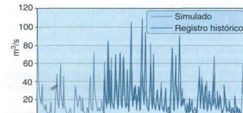
Figura 28. Series mensuales simuladas e históricas del río Tajo en Entrepeñas (periodo 1940-1995)
