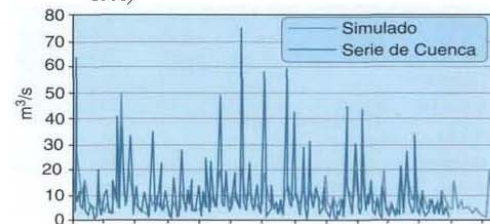
Figura 26. Series mensuales simuladas e históricas del río Segura en Fuensanta (periodo 1940-1995)
