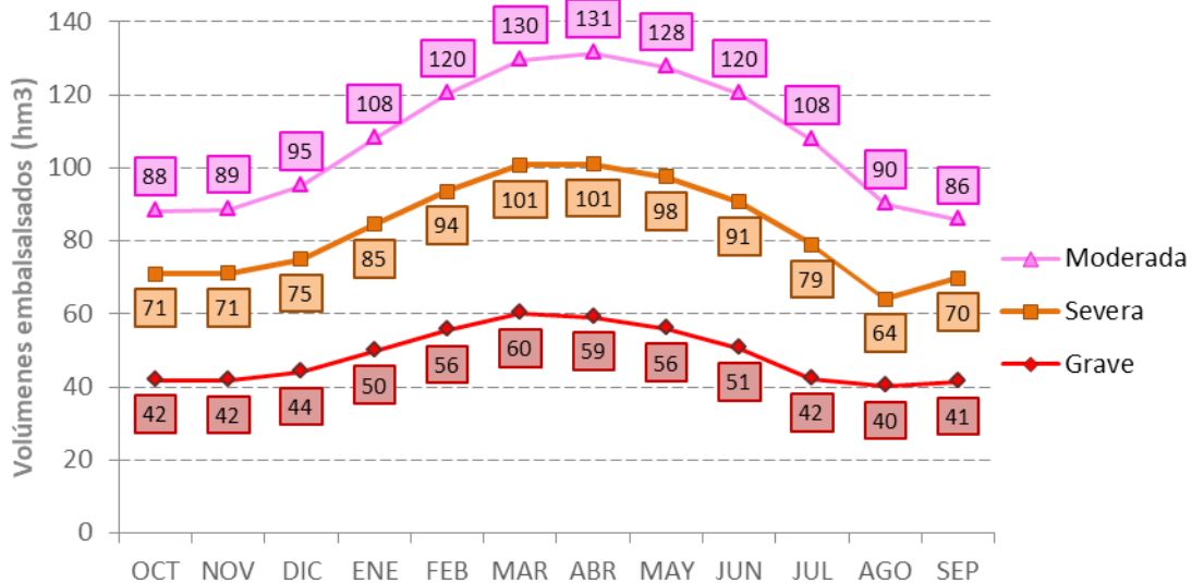
Gráfico 5-20 Umbral de escasez UTE 03 Sistema de Regulación del Barbate
