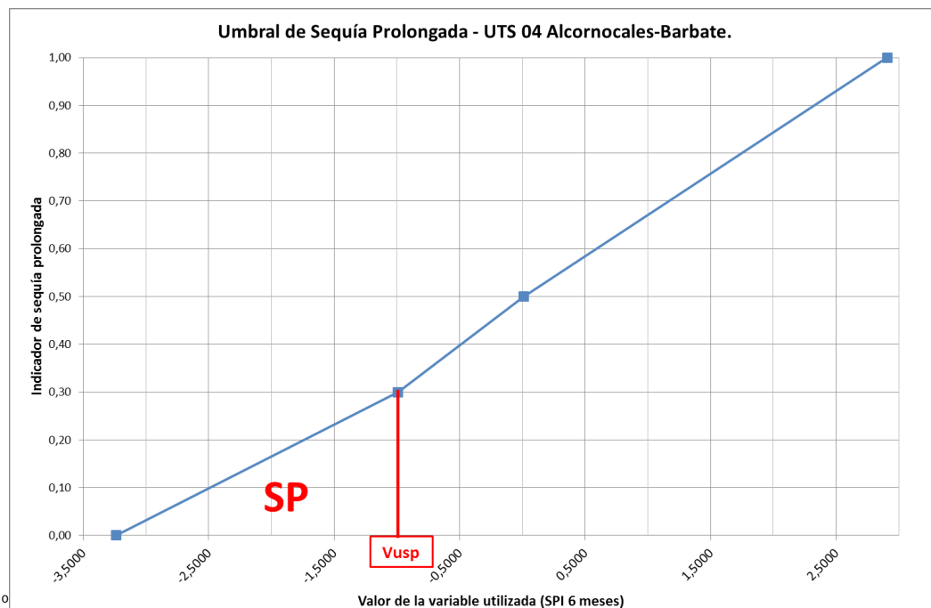
Gráfico 5-8 Umbral de sequía prolongada de la UTS04 - Alcornocales-Barbate.
