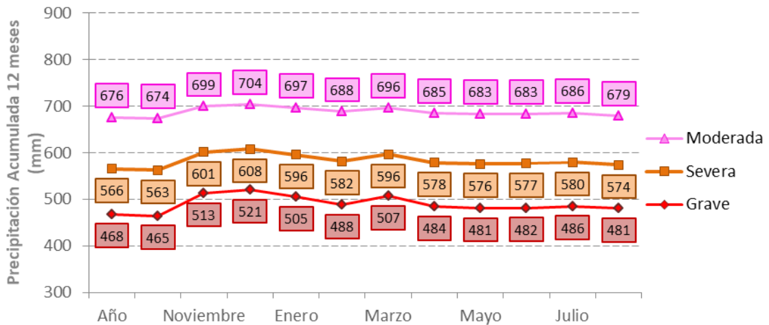
Gráfico 5-14 Umbral de escasez UTE 01 Sierra de Cádiz
