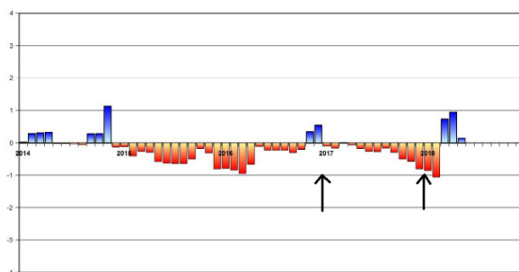
Índice estandarizado de sequía pluviométrica 1950 - 2018 en Andalucía. Detalle de los últimos cinco años.
