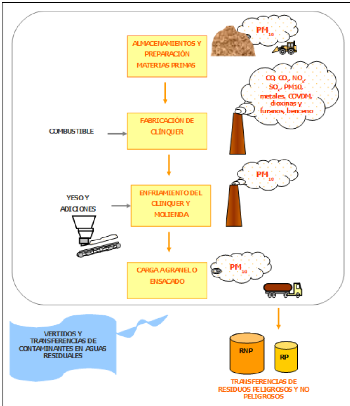
Figura 1. Diagrama de proceso de fabricación y emisiones asociadas
