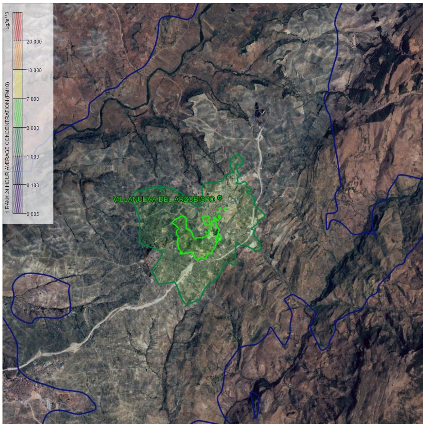
Figura A.18. Contribución máxima diaria a los niveles de inmisión de \text{PM}_{10} Grupo “Calderas de hueso aceituna, orujo y orujillo”
