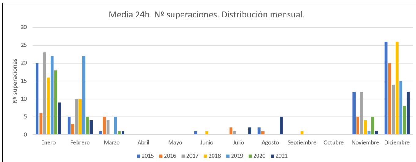
Figura 6.4. Número de superaciones por mes del valor límite diario de PM 10 en el periodo 2015-2021
