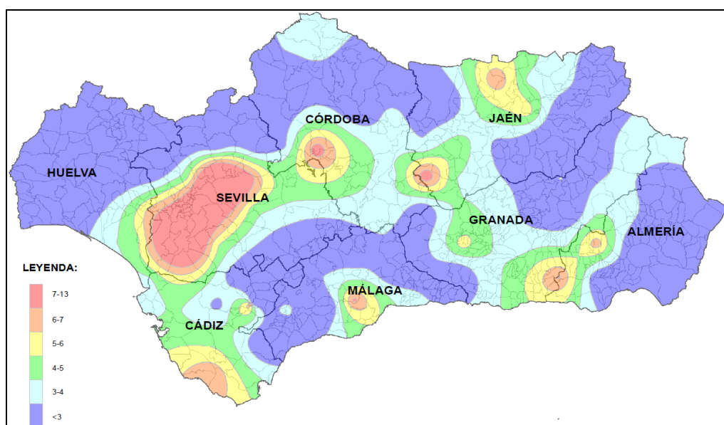
Figura 5.20. Resultados de la campaña de captadores difusivos en fondo rural. Promedio de NO x en 2020
