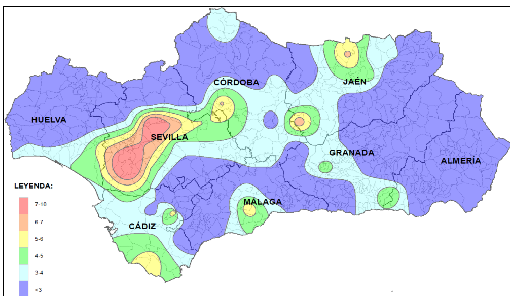
Figura 5.19. Resultados de la campaña de captadores difusivos en fondo rural. Promedio de NO 2 en 2020
