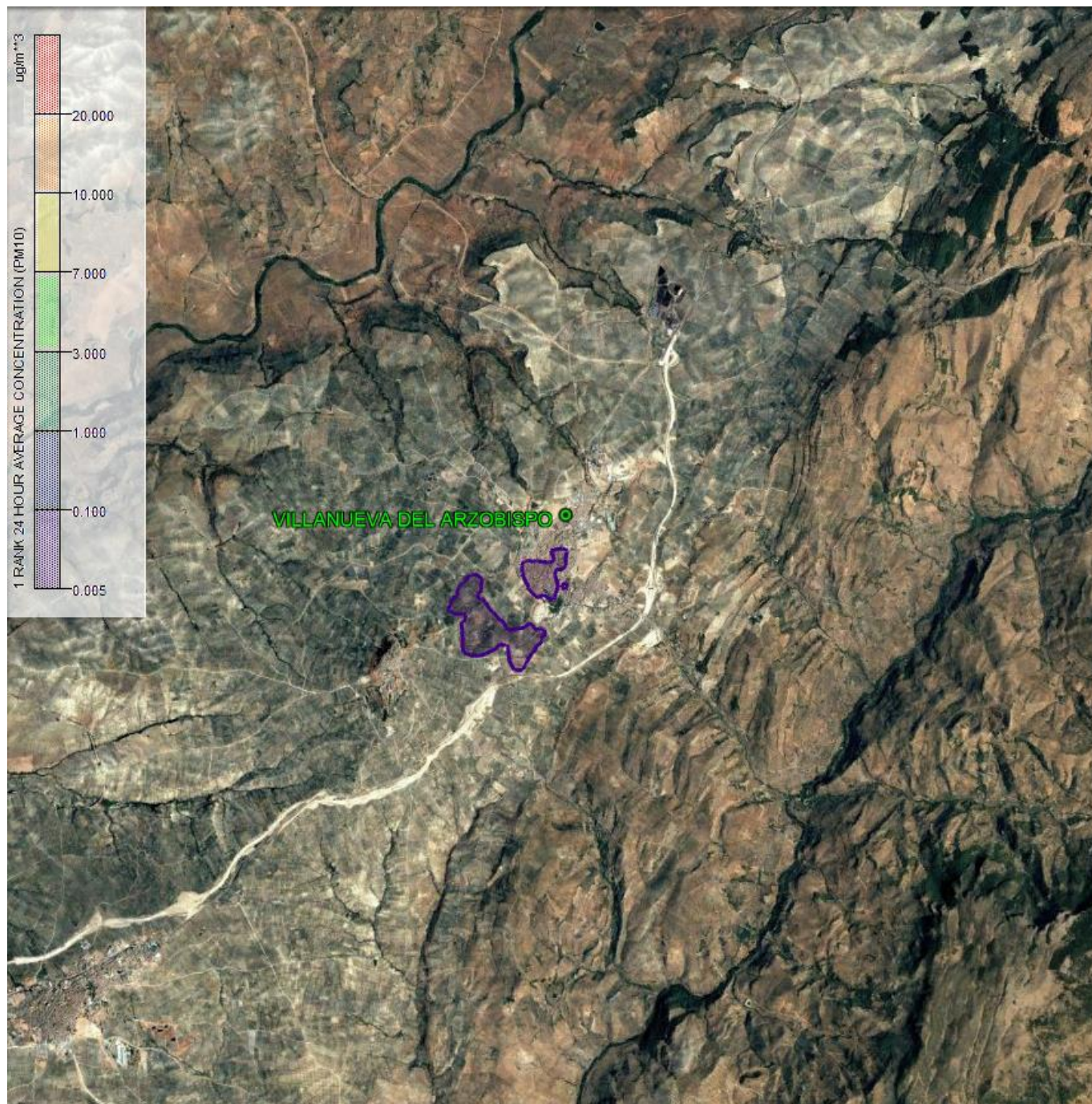
Figura A.24. Contribución máxima diaria a los niveles de inmisión de PM 10 Grupo “Calderas de gas natural”
