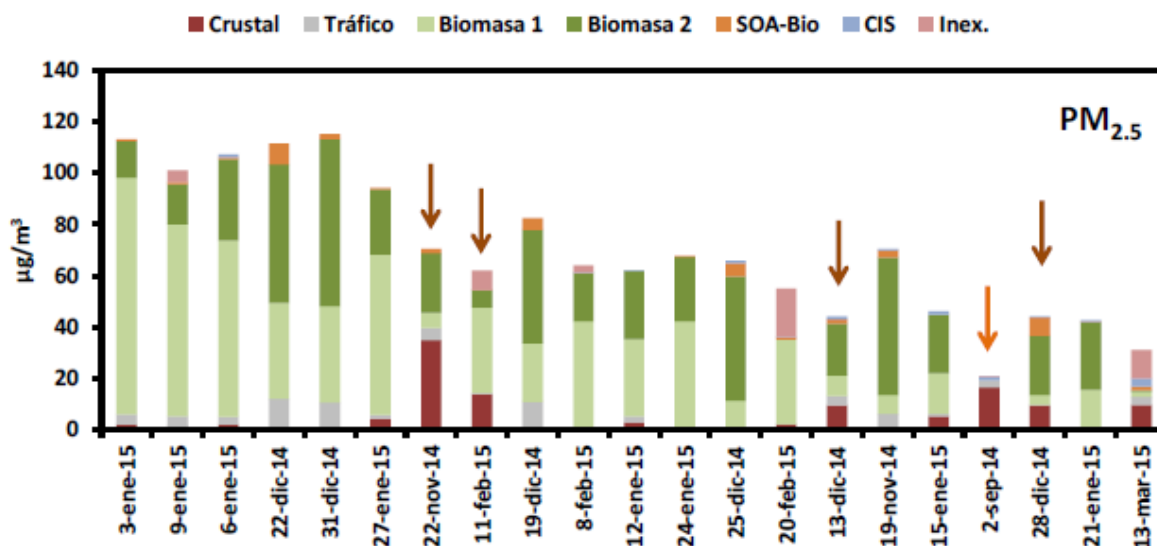
Figura 6.23. Contribución diaria (µg/m 3 ) de las 6 fuentes identificadas a los niveles de PM 2,5 en los días en que se produjeron superaciones del valor límite diario de PM 10
