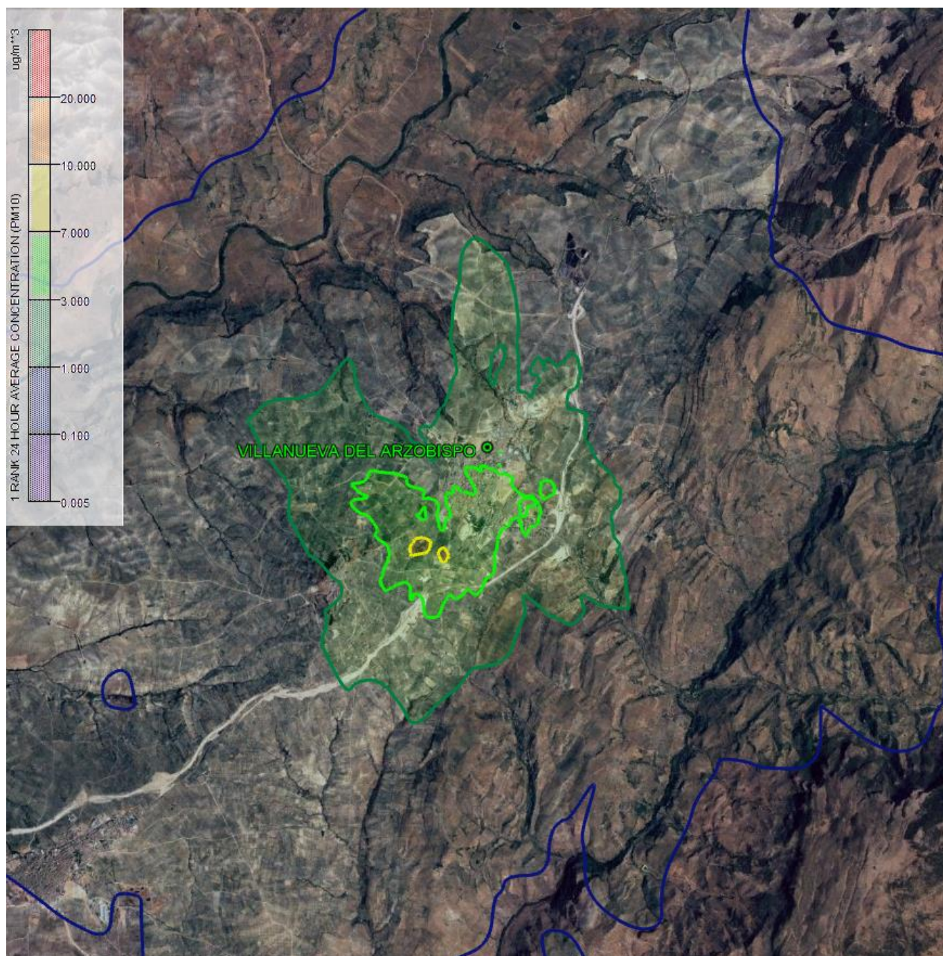
Figura A.19. Contribución máxima diaria a los niveles de inmisión de \text{PM}_{10} Grupo “Calderas de leña y mixtas”
