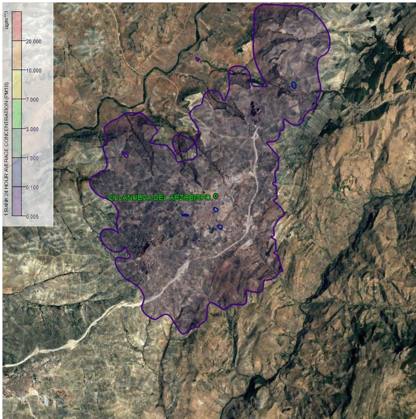
Figura A.23. Contribución máxima diaria a los niveles de inmisión de \text{PM}_{10} Grupo “Estufas de hueso de aceituna y orujillo”
