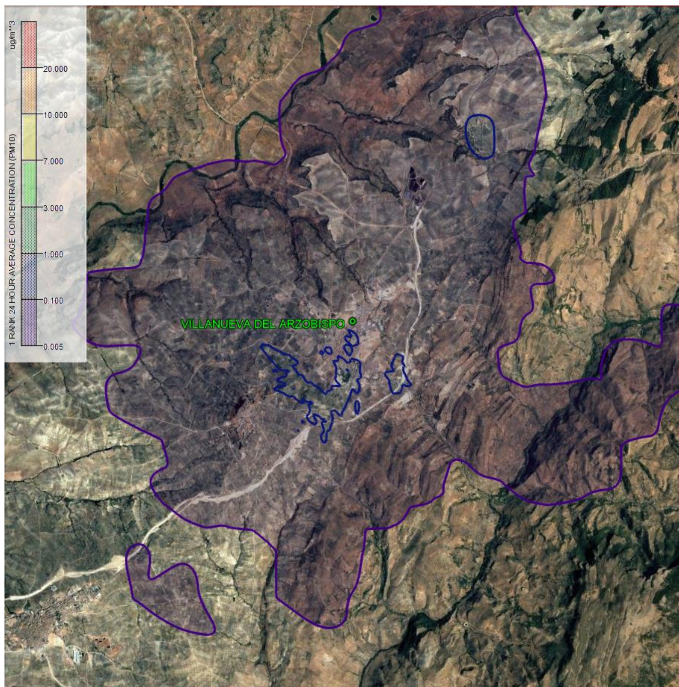
Figura A.20. Contribución máxima diaria a los niveles de inmisión de \text{PM}_{10} Grupo “Calderas de pellets”
