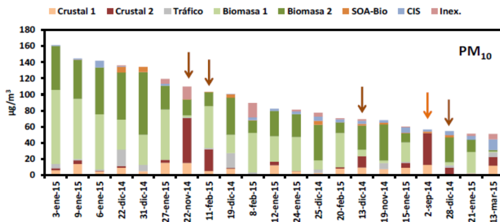
Figura 6.22. Contribución diaria (µg/m 3 ) de las 7 fuentes identificadas a los niveles de PM 10 en los días en que se produjeron superaciones del valor límite diario de PM 10
