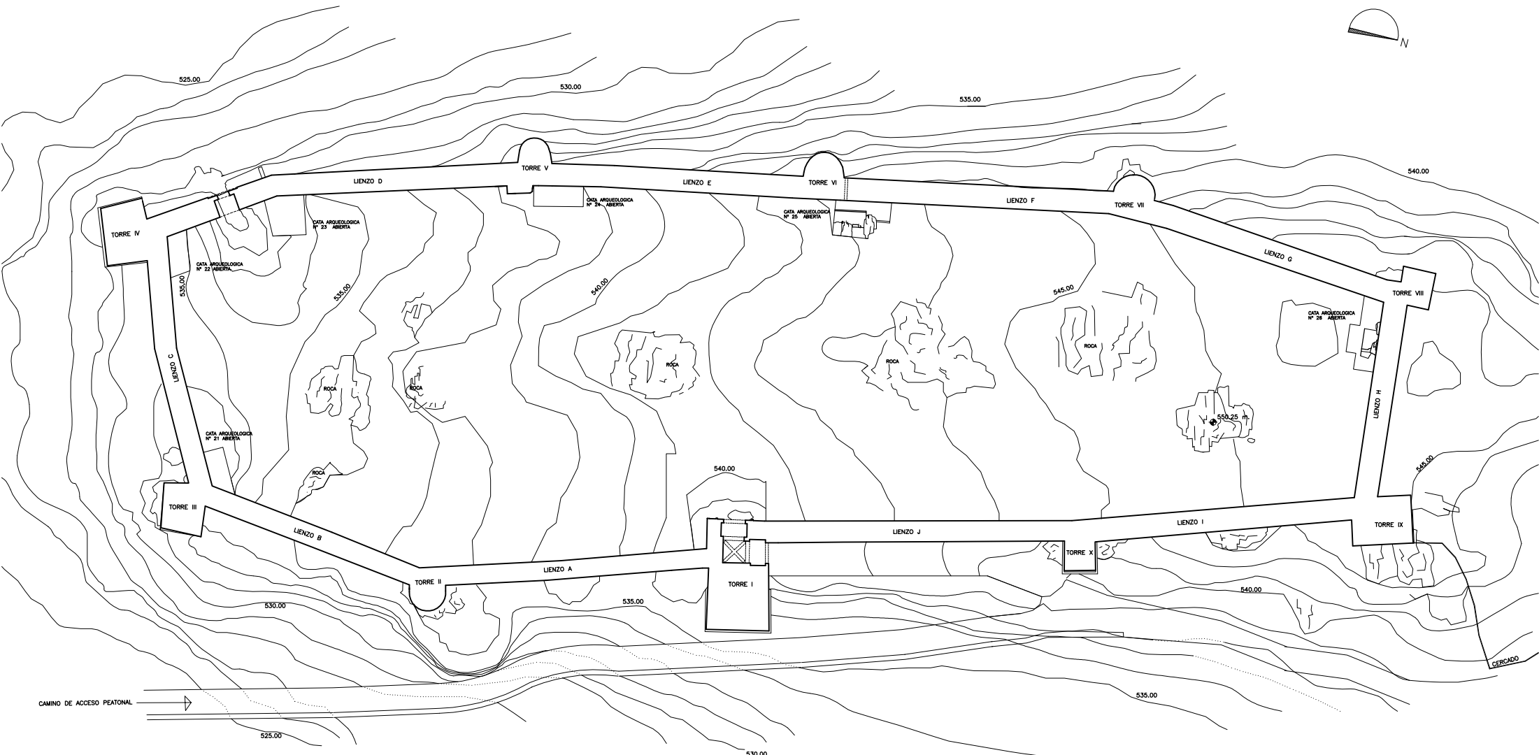
PLANTA GENERAL. TOPOGRAFÍA DEL EMPLAZAMIENTO.
