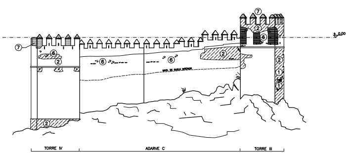
ALZADO SUR
