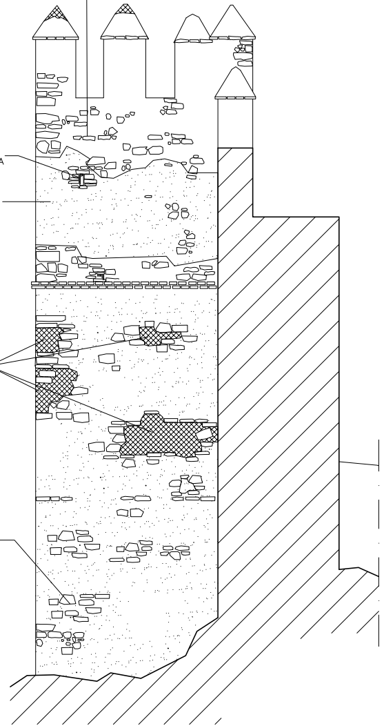
ALZADO NORTE
