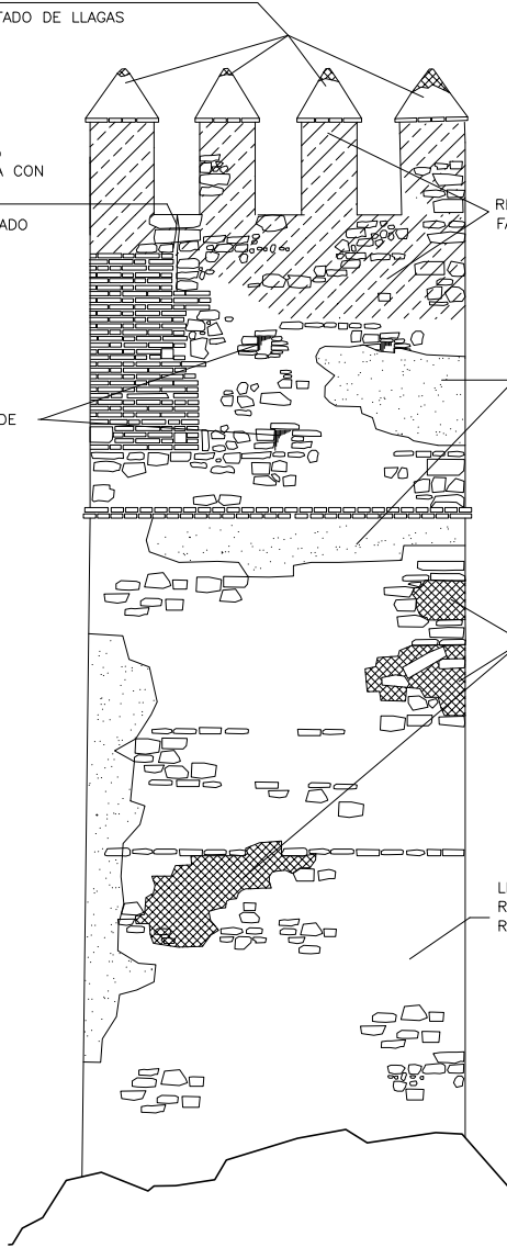
ALZADO ESTE
