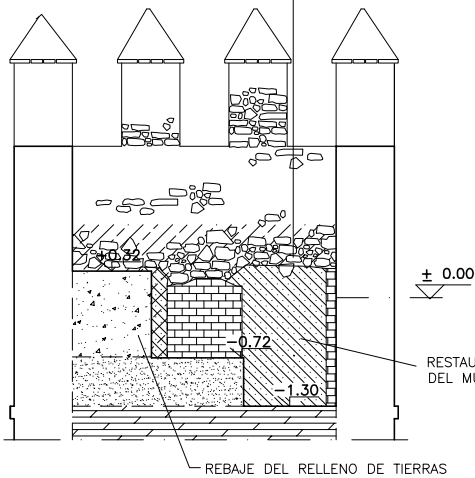
SECCION A-A'
