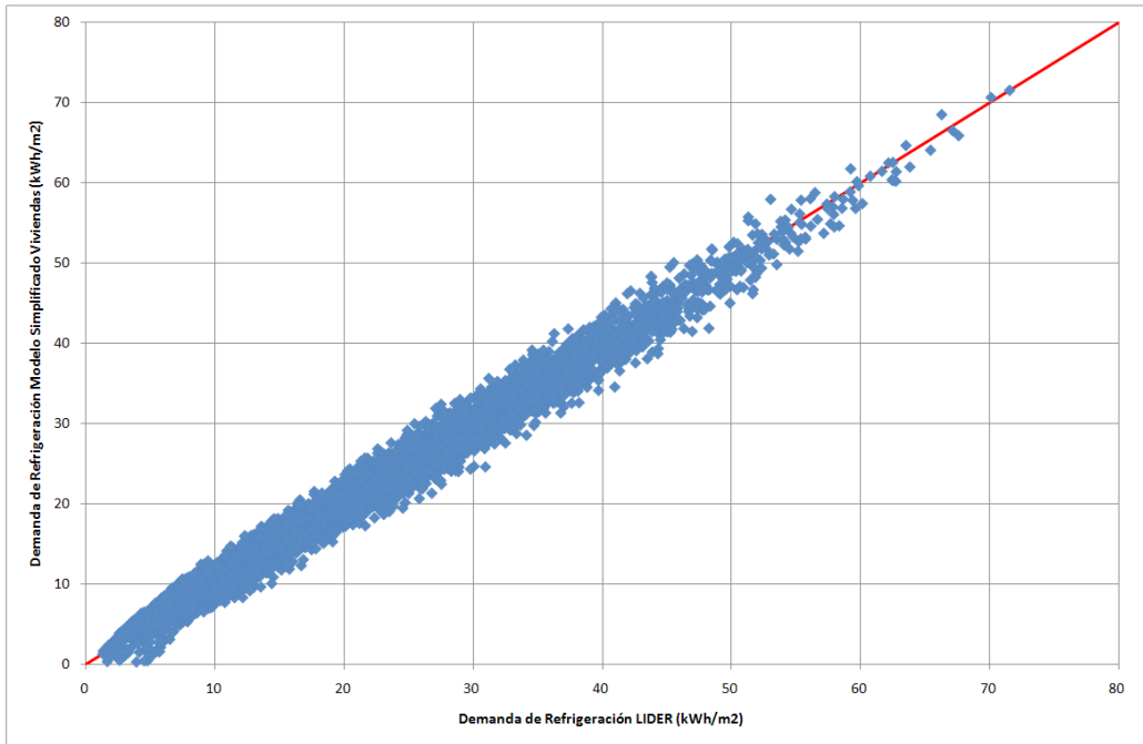
Figura 7. REFRIGERACIÓN. Comparación de los resultados obtenidos aplicando el modelo con las demandas simuladas a través de LIDER.
