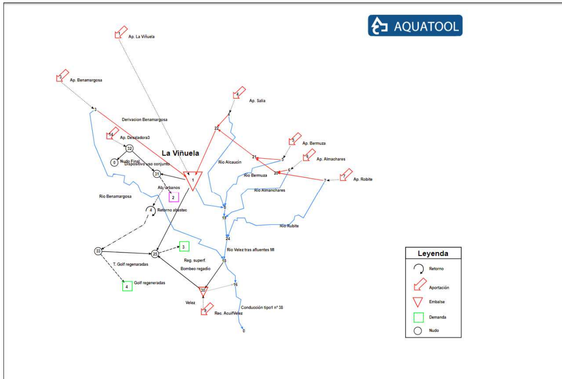
Figura nº 8. Esquema Aquatool del subsistema II-1 en el horizonte 2039
