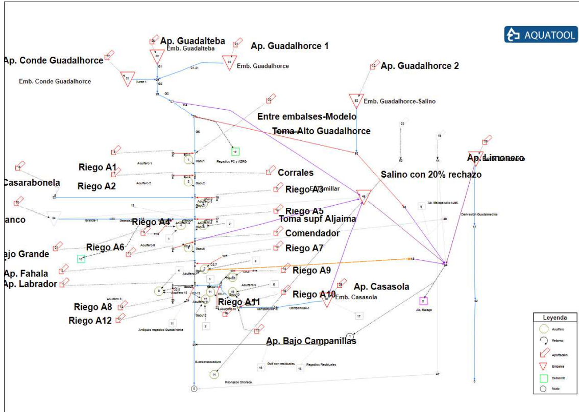
Figura nº 4. Esquema Aquatool del subsistema I-4 en el escenario situación actual y horizonte 2027.
