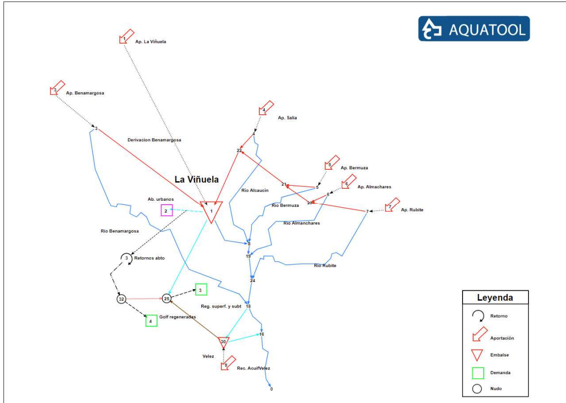
Figura nº 7. Esquema Aquatool del subsistema II-1 en el horizonte 2027
