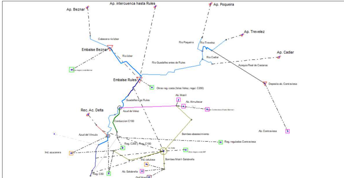
Figura nº 9. Esquema Aquatool del subsistema III-2 en el escenario situación actual.
