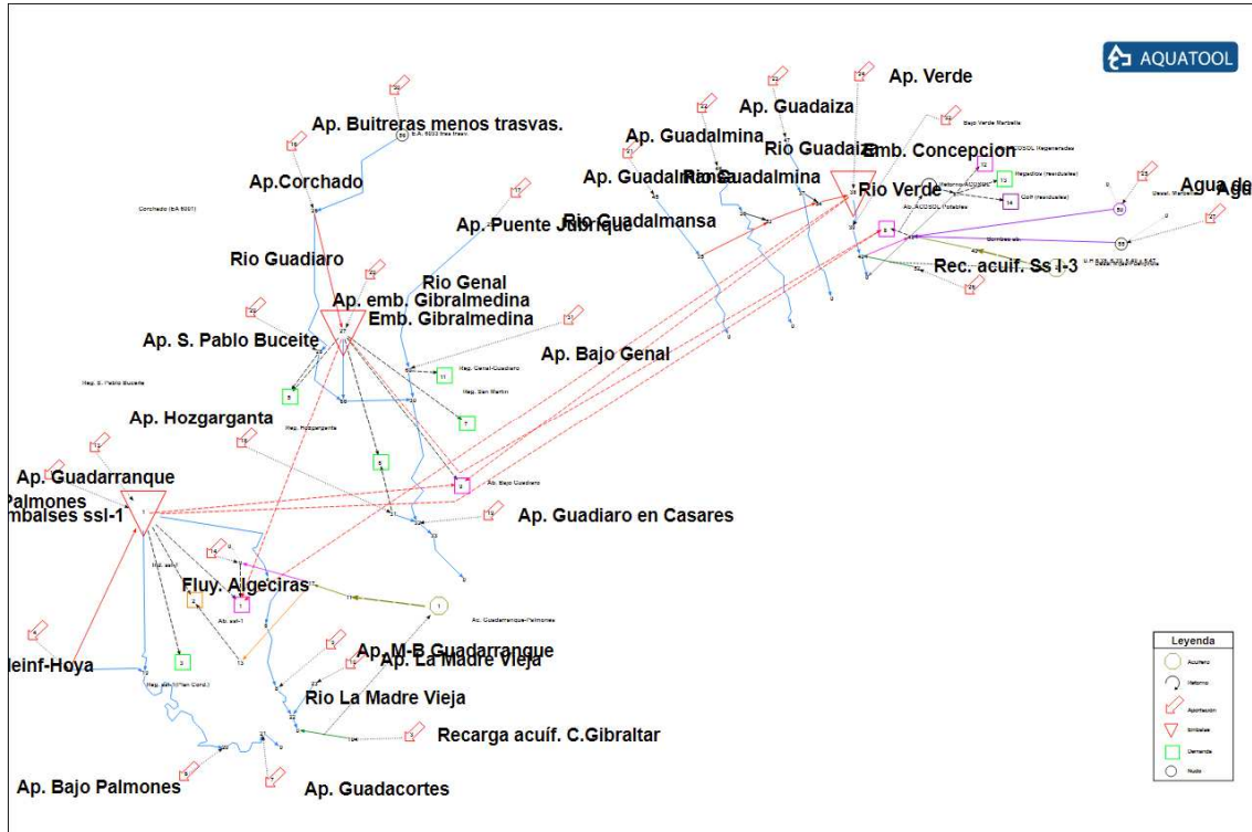
Figura nº 3. Esquema Aquatool de los subsistemas I-1, I-2 y I-3 en el horizonte 2039
