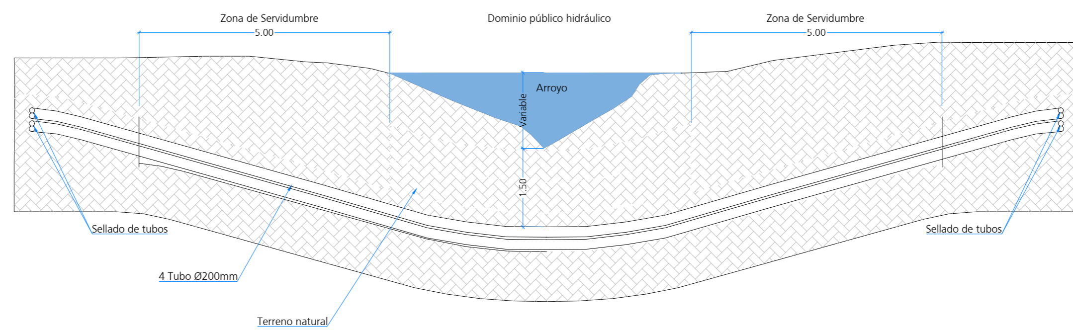
Sección longitudinal cruce de arroyo. Perforación horizontal dirigida Esc: S/E
