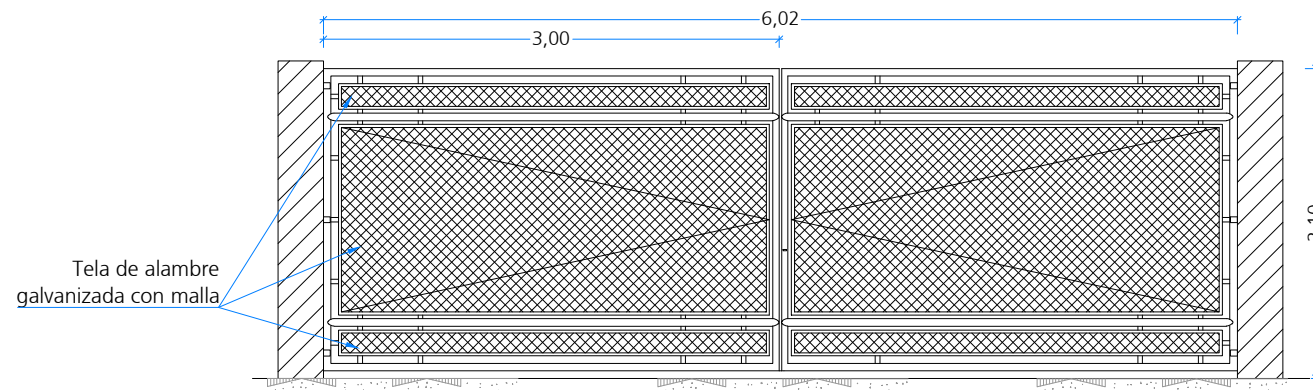
Puerta acceso vehiculos. Vista frontal
