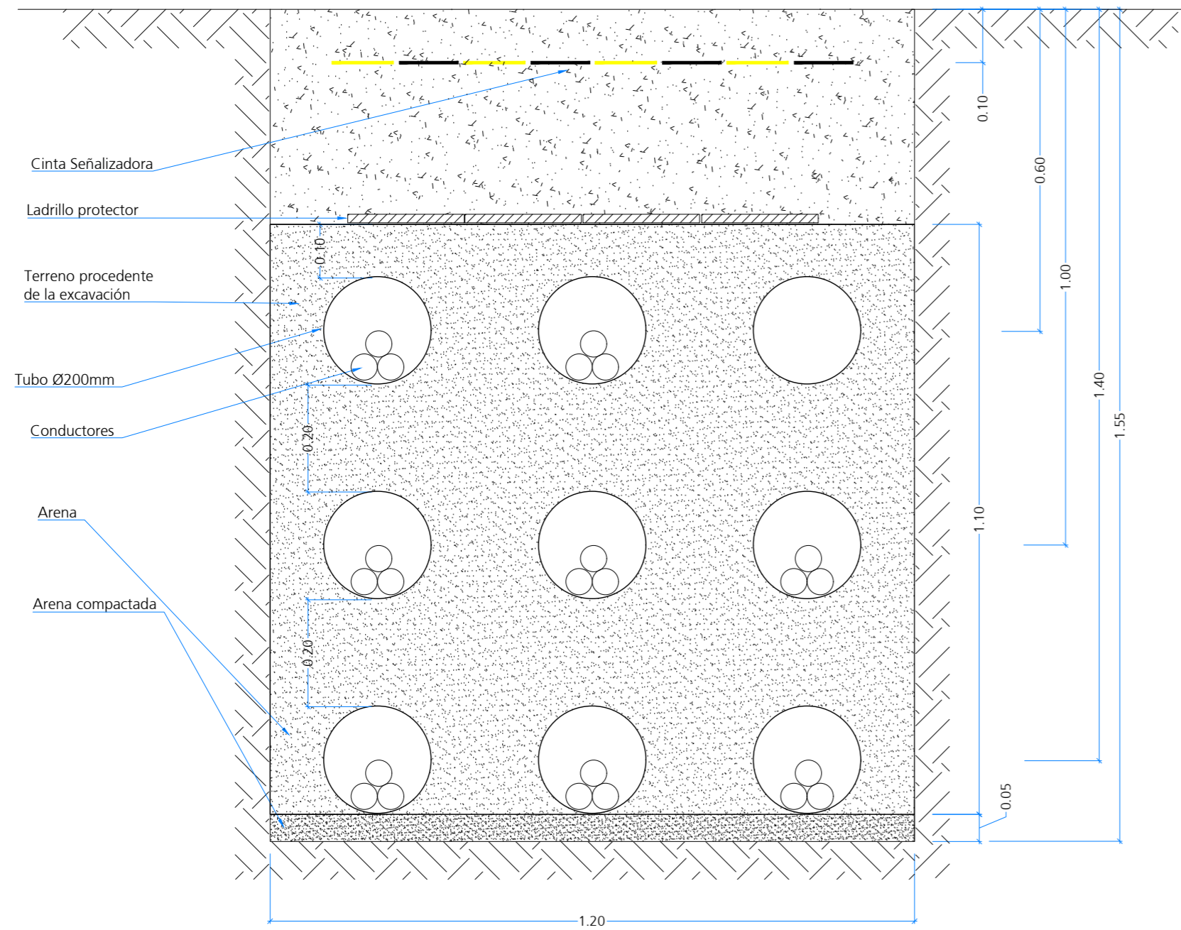
LSMT (45kV) Evacuación general común subterránea (4x) hacia SET Promotores Pinar de Rey
