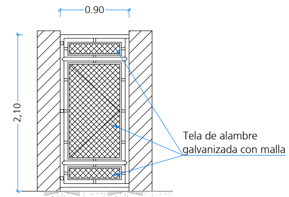
Puerta acceso personas. Vista frontal
