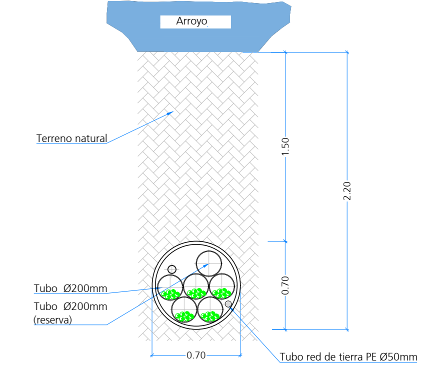
Sección tipo cruce de arroyo. Perforación horizontal dirigida Esc: S/E
