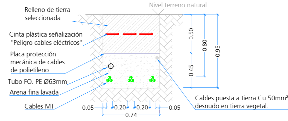
Zanja tipo 11 Zanja 3 CTOs. MT
