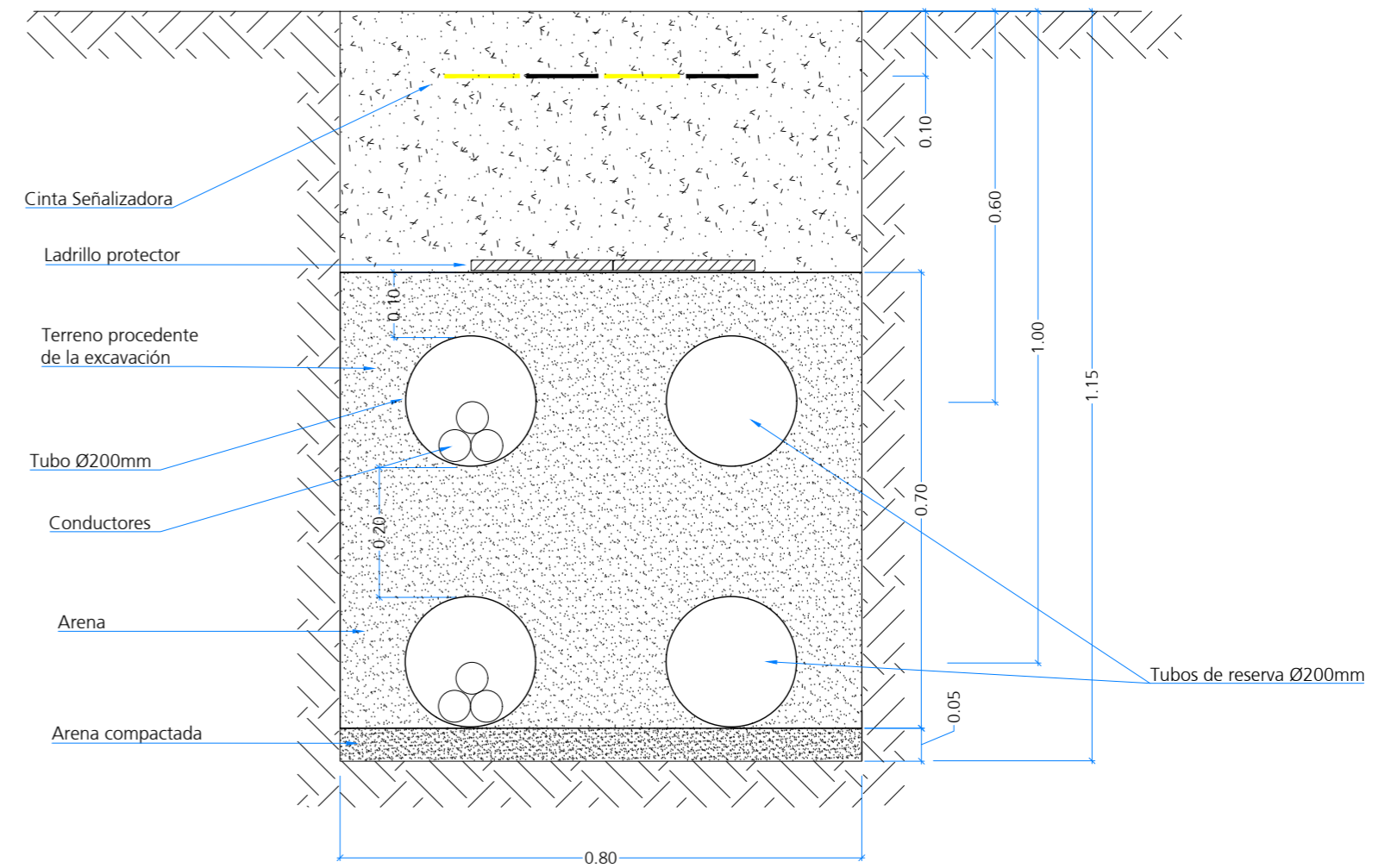
LSMT (45kV) desde CS (FV Mitralax Pto Sta. María) hacia SET Promotores Pinar de Rey
