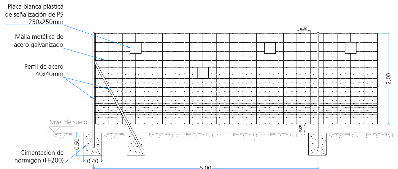
Vallado tipo cinégetico. Vista frontal
