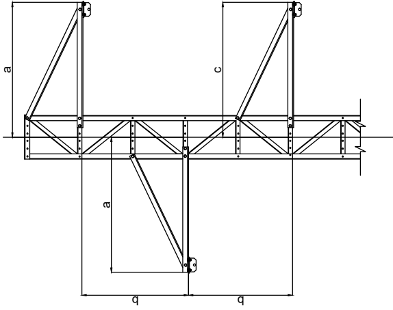
ARMADO TRESBOLILLO PARA APOYOS CELOSÍA
