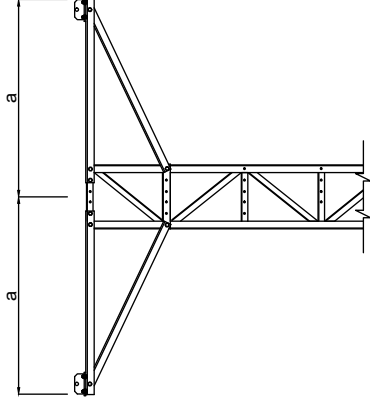
ARMADO MO PARA APOYOS CELOSÍA
