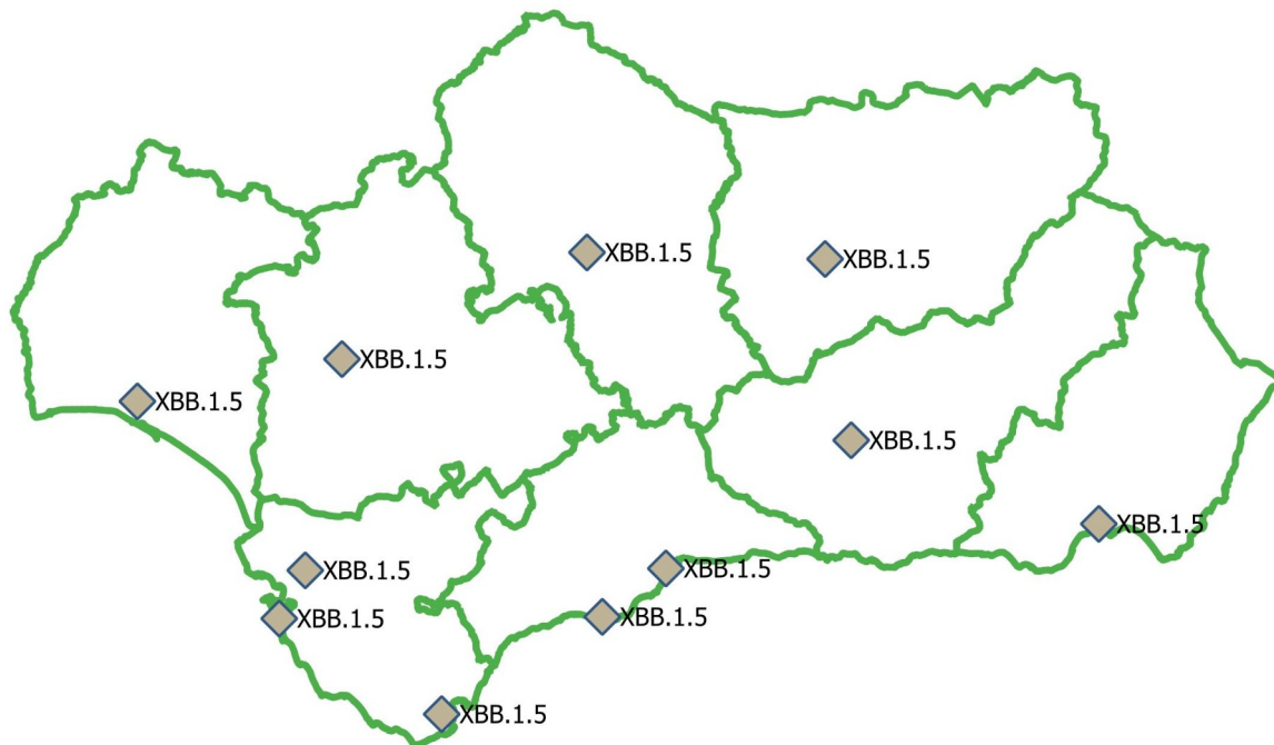
Figura 3. Variante detectada en mayor proporción en los distintos territorios en el análisis de secuenciación mensual. MAYO 2023.
