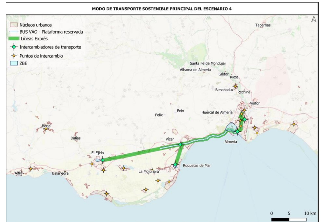
Ilustración 19. Actuaciones consideradas en el Escenario 4
